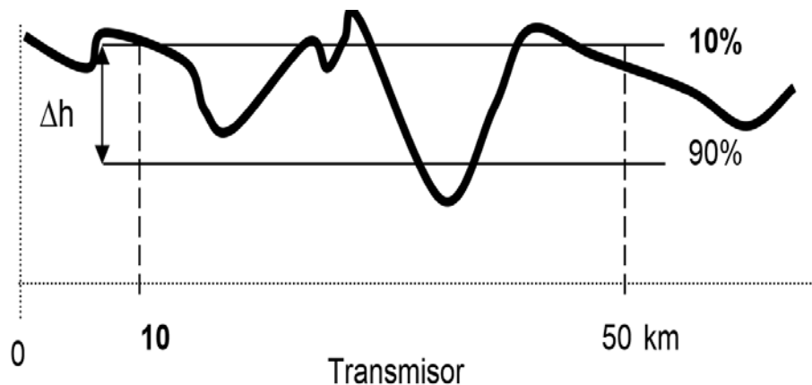
FIGURA 04 GRÁFICA DE IRREGULARIDAD DEL TERRENO
