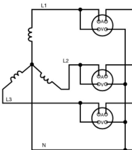
3 FASES, 4 HILOS, 3 ELEMENTOS
