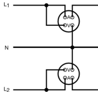
MONOFÁSICO 3 HILOS DOS ELEMENTOS
