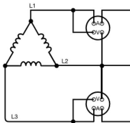
3 FASES, 3 HILOS, 2 ELEMENTOS
