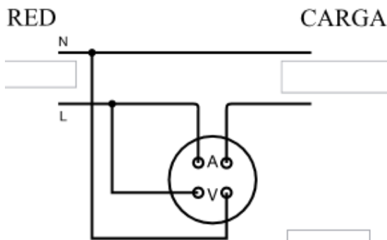
MONOFÁSICO 2 HILOS
