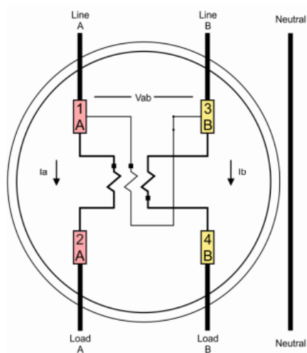
MEDIDOR TIPO 2S CFE
