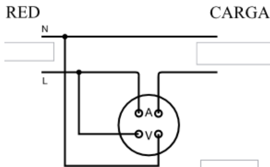
MONOFÁSICO 2 HILOS
