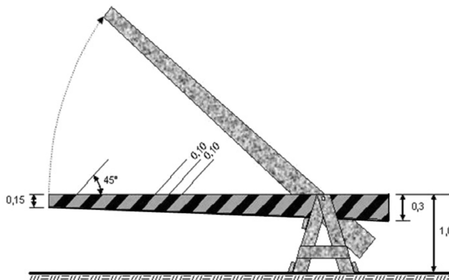
FIGURA 2.- Barrera levadiza
