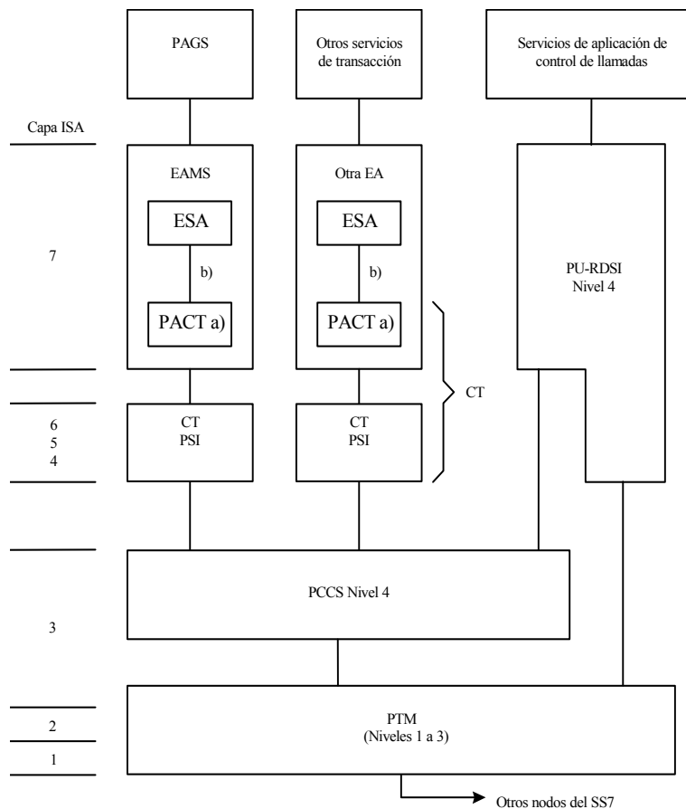
FIGURA 5.- Relación entre los niveles funcionales del SS7 y la estructura de capas ISA.
