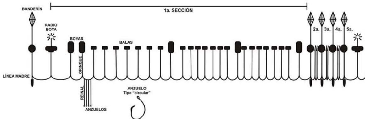
Figura 23. Esquema del arete de pesca "palangre" utilizado para la pesca del atún aleta amarilla ( Thunnus albacares ) en el Golfo de México, durante 2005. El esquema fue diseñado en base a la información proporcionada por el PNAAPD a través de su Programa de Observadores a bordo.
