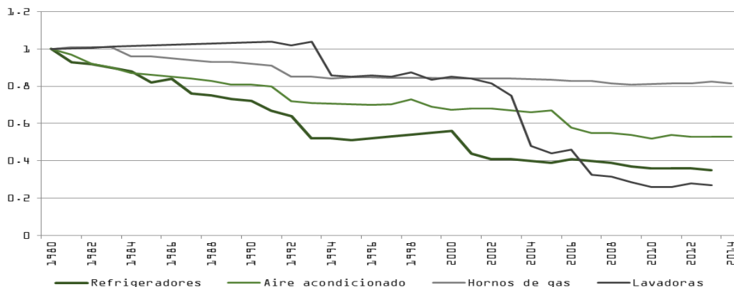
FIGURA 9. CONSUMO DE ENERGÍA PROMEDIO DE NUEVOS ELECTRODOMÉSTICOS VENDIDOS EN EL PERIODO 1980 – 2014 (Índice base 1980)
