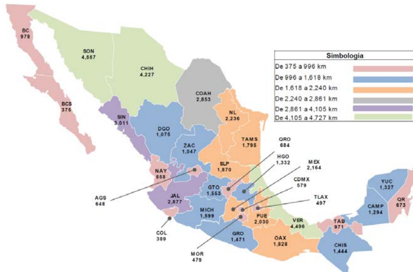
FIGURA 14. LONGITUD DE LÍNEAS DE TRANSMISIÓN (230 Y 400 KV) POR ENTIDAD FEDERATIVA
