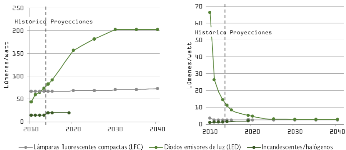
FIGURA 7. EFICIENCIA PROMEDIO EN ILUMINACIÓN (PRODUCCIÓN DE LUZ POR UNIDAD DE ENERGÍA CONSUMIDA) Y COSTOS POR LÁMPARA
