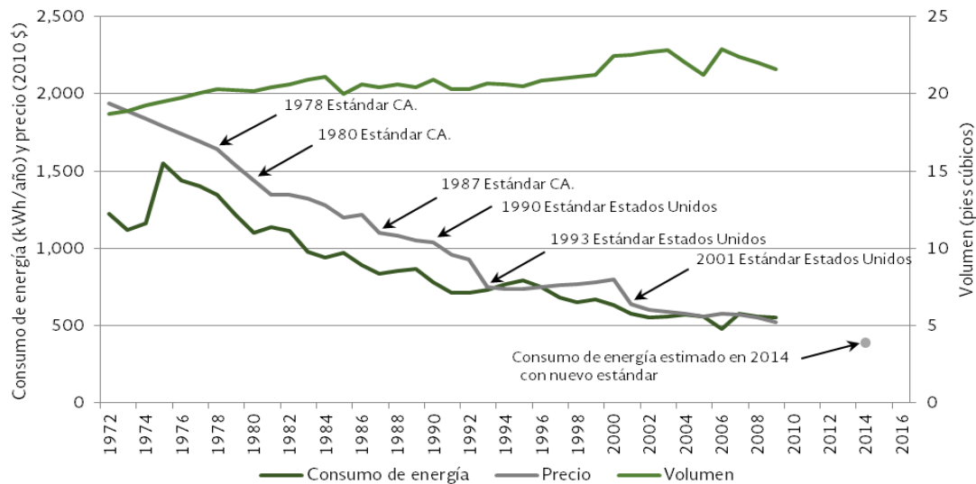
FIGURA 8. CONSUMO PROMEDIO DE ENERGÍA DE REFRIGERADORES RESIDENCIALES, VOLUMEN, Y EVOLUCIÓN DE PRECIO
