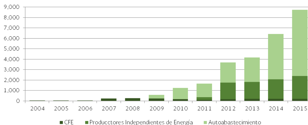
FIGURA 21. EVOLUCIÓN DE LA GENERACIÓN EÓLOELÉCTRICA 2004-2015 (Gigawatts-hora)
