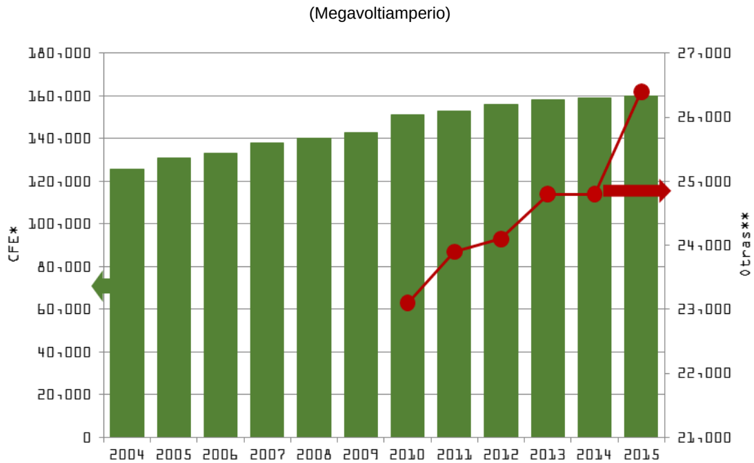
FIGURA 15. CAPACIDAD De SUBESTACIONES, 2004-2015
