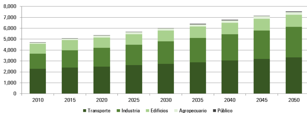
FIGURA 27. CONSUMO FINAL ENERGÉTICO TOTAL POR SECTOR ESCENARIO BASE, 2016-2050 (Petajoules)
