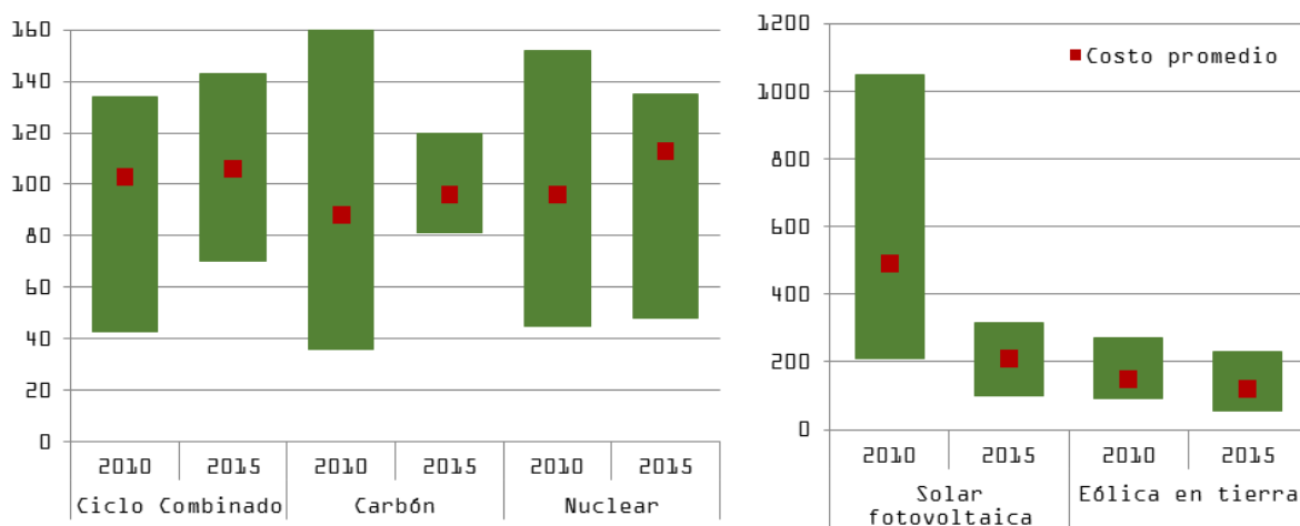
FIGURA 3. COSTOS NIVELADOS DE ENERGÍAS FÓSILES Y RENOVABLES ENTRE 2010 Y 2015 (USD/MWH)
