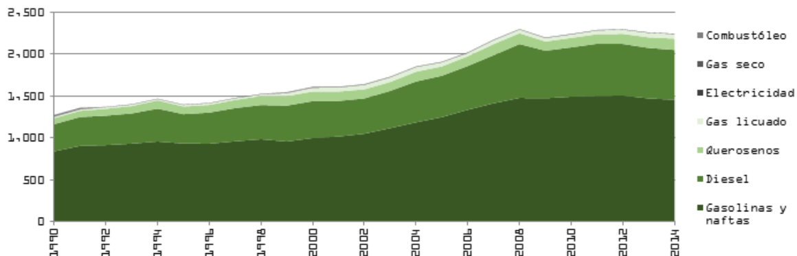
FIGURA 19. CONSUMO DE COMBUSTIBLES DEL SECTOR TRANSPORTE (Petajoules)
