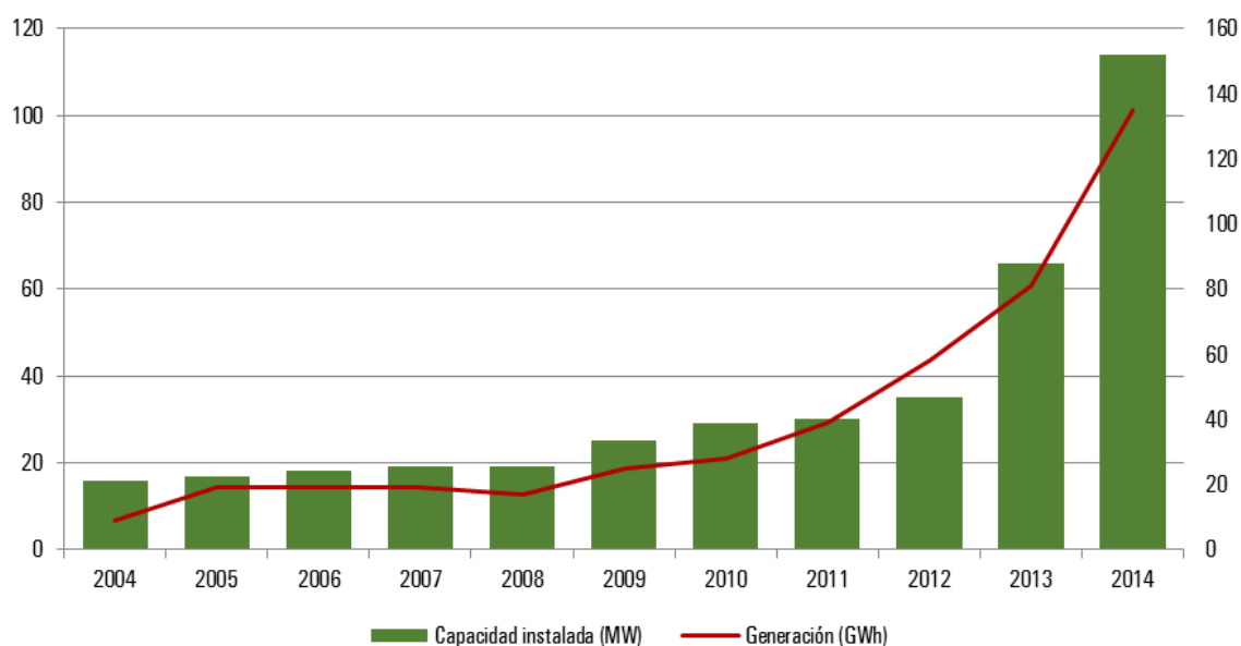
FIGURA 22. EVOLUCIÓN DE LA ENERGÍA FOTOVOLTAICA 2004-2015
