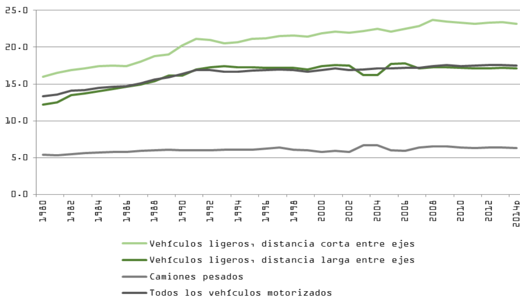
FIGURA 6. RENDIMIENTO PROMEDIO DE VEHÍCULOS EN ESTADOS UNIDOS 1980 – 2014 (Millas por galón)
