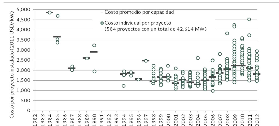
FIGURA 4. COSTOS DE INSTALACIÓN DE PROYECTOS EÓLICOS EN LOS ESTADOS UNIDOS, 1982 - 2012
