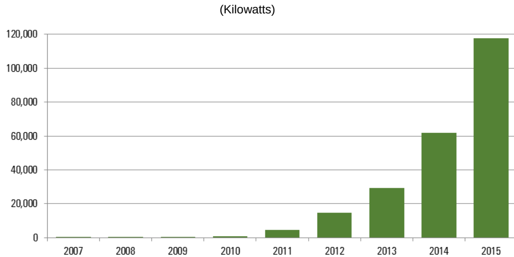
FIGURA 23. EVOLUCIÓN DE LA CAPACIDAD INSTALADA POR CONTRATOS DE INTERCONEXIÓN DE PEQUEÑA Y MEDIANA ESCALA 2007-2015
