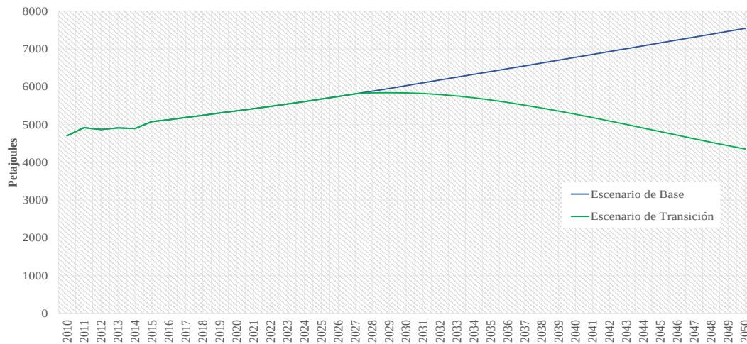
FIGURA 33. COMPARACIÓN DEL CONSUMO FINAL ENERGÉTICO, 2016-2050 (Petajoules)
