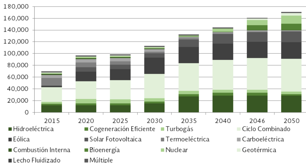
FIGURA 29. CAPACIDAD INSTALADA DE GENERACIÓN DE ELECTRICIDAD, 2015-2050
