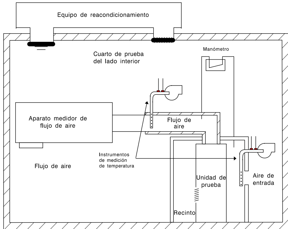
FIGURA 3. Calorímetro aire-entalpía
