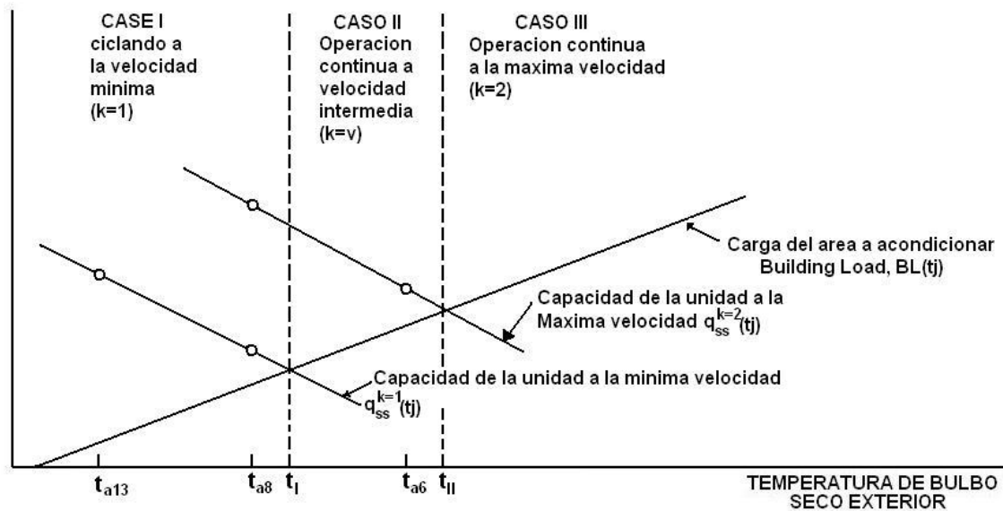
Diagrama esquemático de varios modos de operación para la unidad en modo frío
