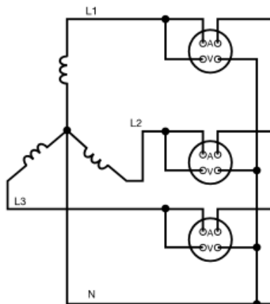
3 FASES, 4 HILOS, 3 ELEMENTOS
