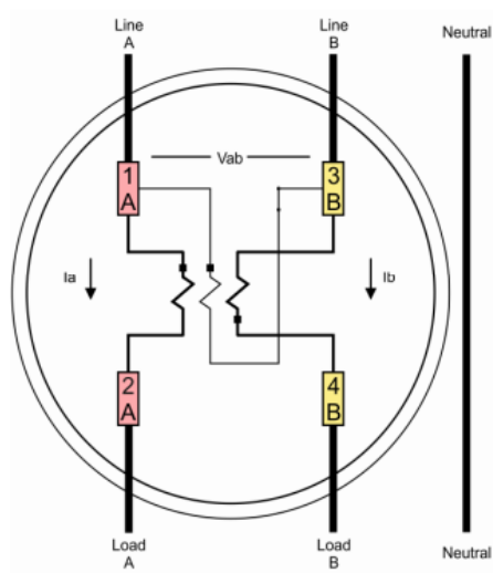
MEDIDOR TIPO 2S CFE
