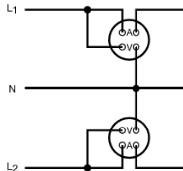
MONOFÁSICO 3 HILOS DOS ELEMENTOS
