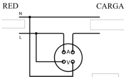
MONOFÁSICO 2 HILOS
