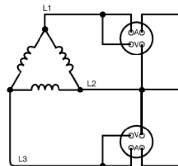
3 FASES, 3 HILOS, 2 ELEMENTOS
