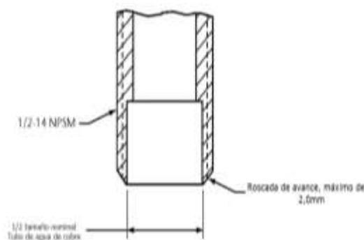
Figura 2. Dimensiones para conectores macho 1/2- 14 NPSM
