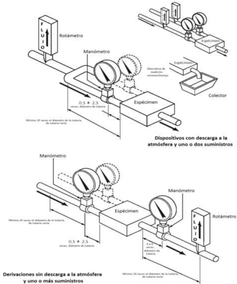
Figura 4.- Banco de pruebas para determinar el gasto mínimo y máximo de un espécimen.
