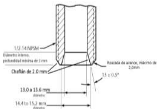
Figura 2. Dimensiones para conectores macho 1/2- 14 NPSM
