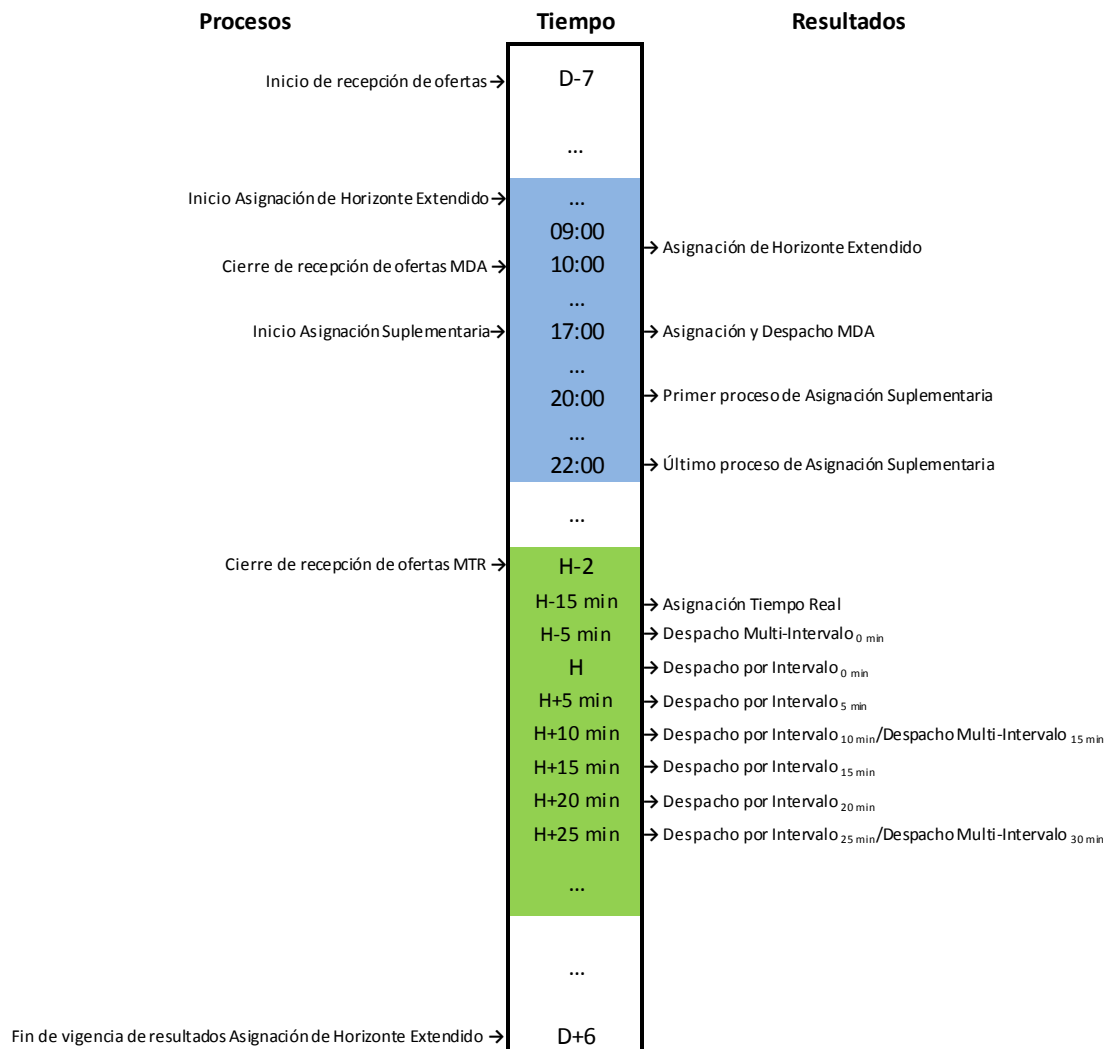
Figura 1. Cronograma de procesos para el Mercado de Energía de Corto Plazo.
