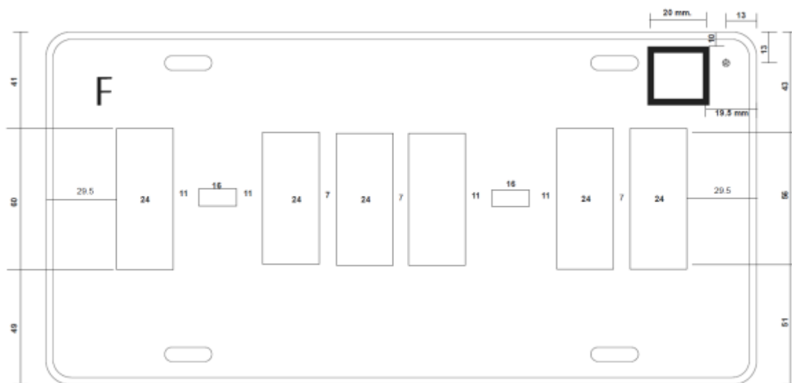
Figura 3 Para vehículos del Servicio de Autotransporte Federal Transfronterizo de pasaje. Separación de caracteres (letras y dígitos), placas con seis caracteres y guiones. Acotaciones en milímetros. El ancho de los caracteres debe ser de acuerdo a lo indicado en la figura. Las dimensiones de los guiones serán de 16 x 5.6. Se incorporará la letra "T" y "F" según corresponda a la placa.
