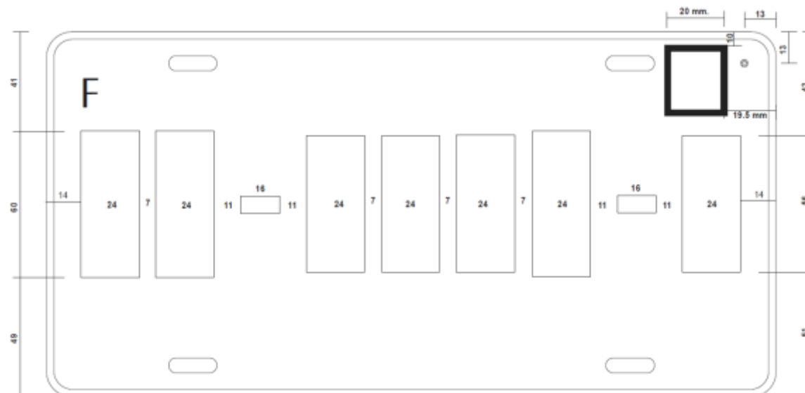
Figura 10 Para vehículos de corporaciones policiacas y de vigilancia Separación de caracteres (letras y dígitos), placas con siete caracteres y guiones. Acotaciones en milímetros.
