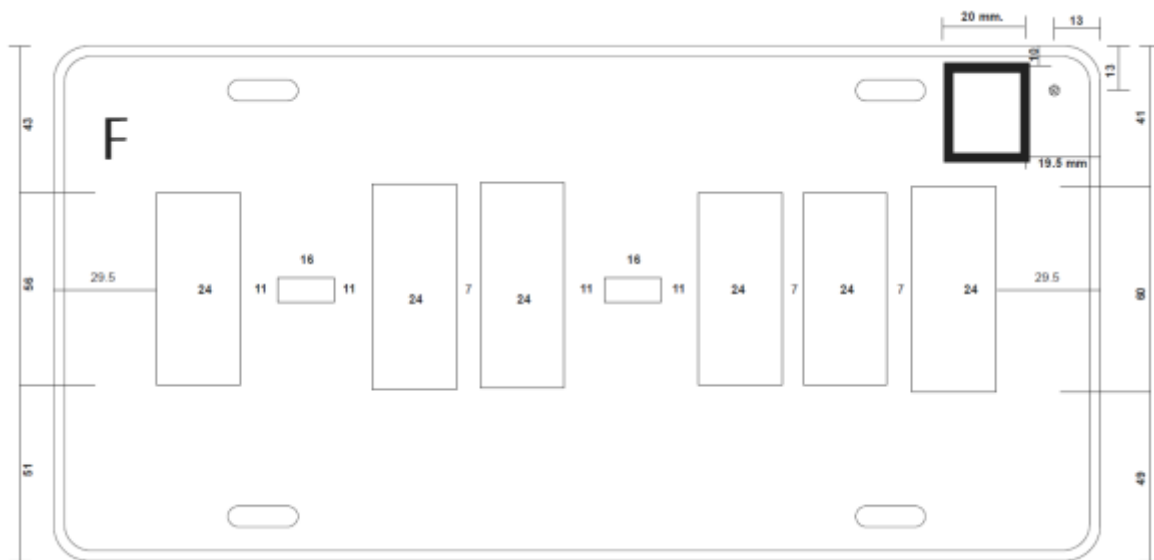
Figura 13 Para Vehículos de Demostración para las Entidades Federativas Separación de caracteres (letras y dígitos), placas con seis caracteres. Acotaciones en milímetros. El ancho de los caracteres debe ser de acuerdo a lo indicado en la figura. Las dimensiones de los guiones serán de 16 x 5.6. Se incorporará la letra "T" y "F" según corresponda a la placa.
