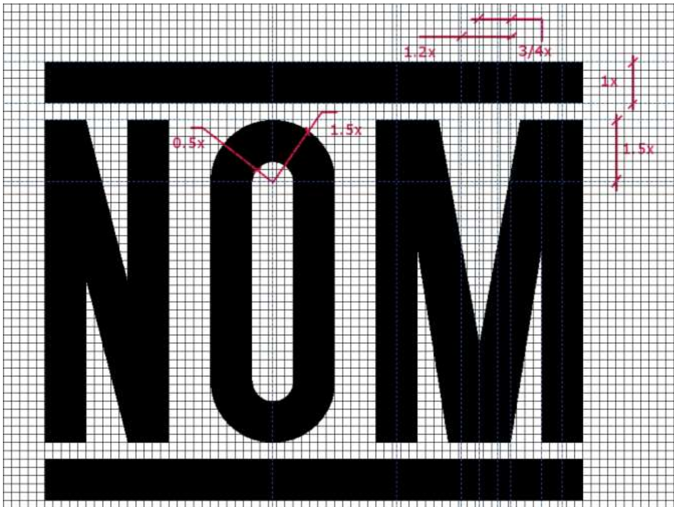
Figura A.2 – Trazos de la Contraseña Oficial NOM.
