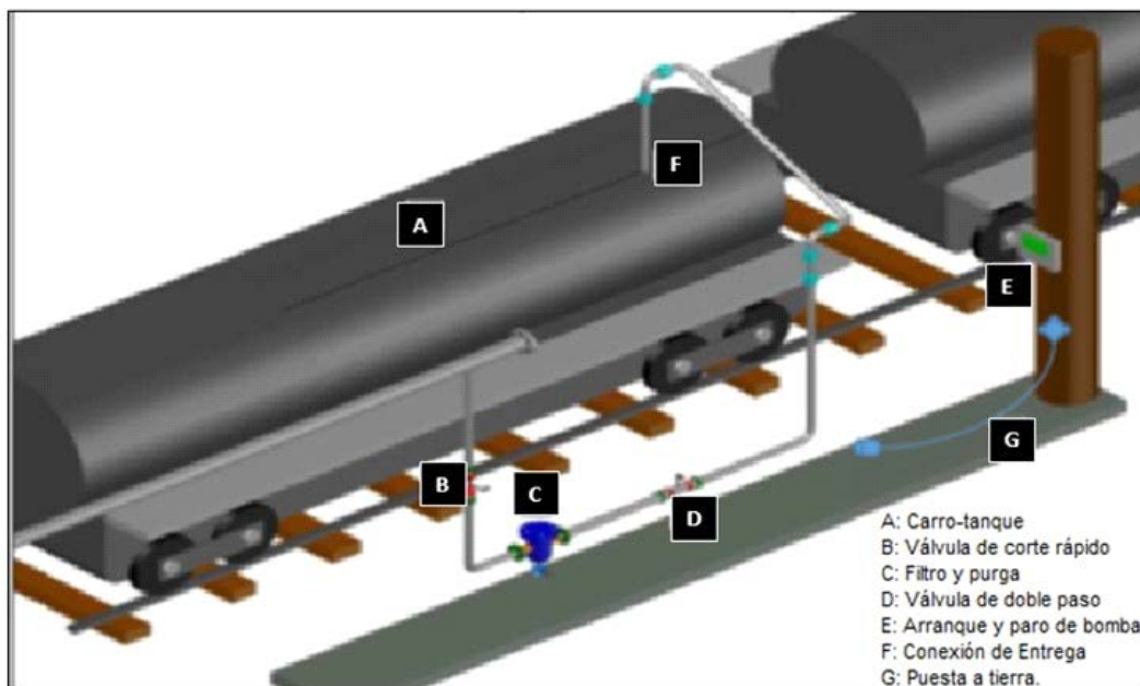
Figura 4. Sistema de Recepción de Carro-tanque.
