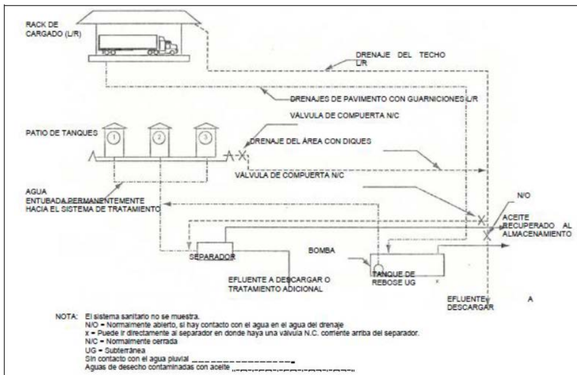
Figura 7. Drenaje pluvial y aceitoso.
