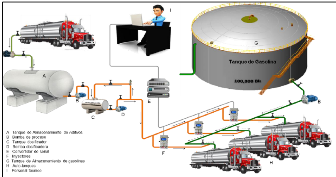
Figura 1. Sistema automático de dosificación de aditivos.
