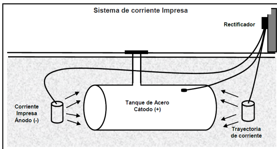
Figura 2B. Sistema de protección catódica por corriente impresa.
