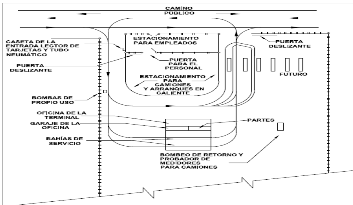
Figura 9. Distribución de patio de carga de Auto-tanques con estacionamiento interno.
