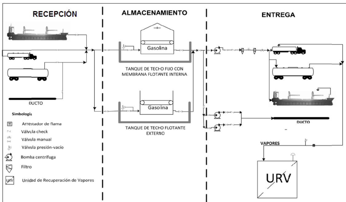
Figura 1A. Almacenamiento, Recepción y Entrega de Gasolinas.
