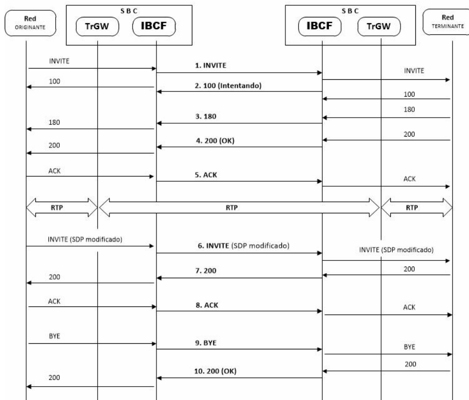
Diagrama 4. Actualización del medio.
