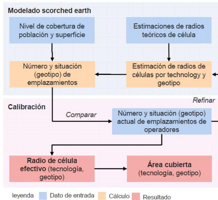
Figura 5: Esquema de modelado scorched earth calibrado para el operador móvil [Fuente: Analysys Mason, 2012]
