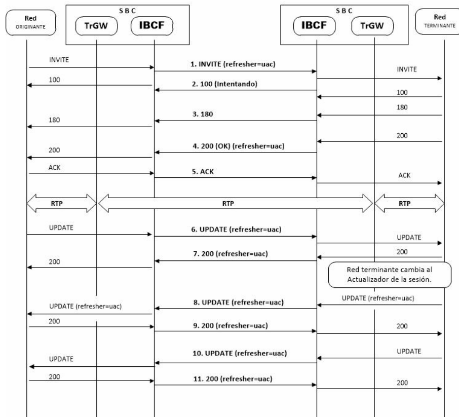
Diagrama 3. Actualización de sesión.
