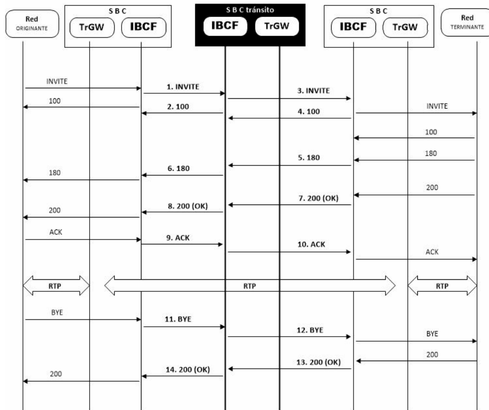
Diagrama 5. Establecimiento de una llamada de tránsito.
