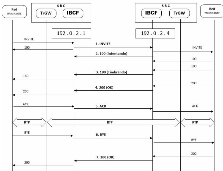
Diagrama 1. Establecimiento de una llamada básica.
