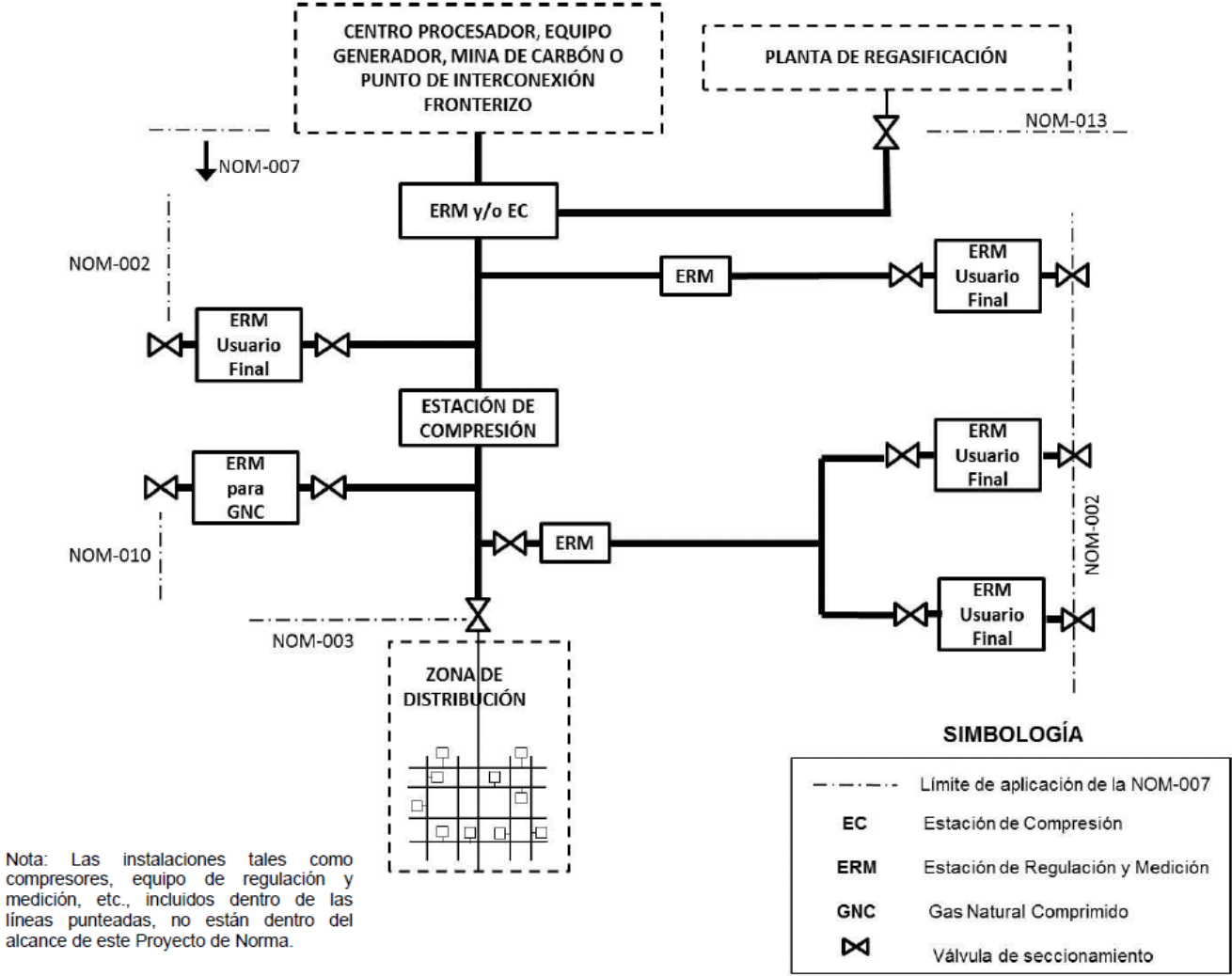
Diagrama 1: Instalaciones de un sistema de transporte que están dentro del alcance de este Proyecto de Norma.
