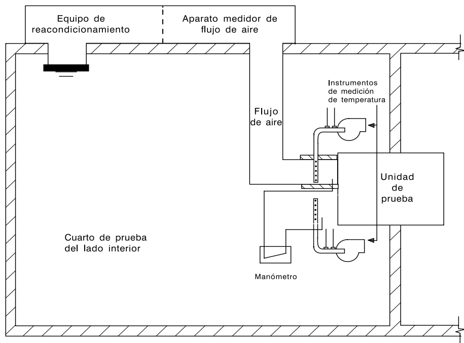
Figura A.4 - Cuarto de aire-entalpía
