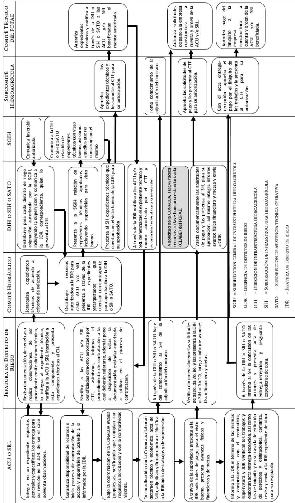
DIAGRAMA DE FLUJO DE LAS ACCIONES DE LA COMPONENTE REHABILITACIÓN, MODERNIZACIÓN Y TECNIFICACIÓN DE DISTRITOS DE RIEGO MODALIDA FOFAE
