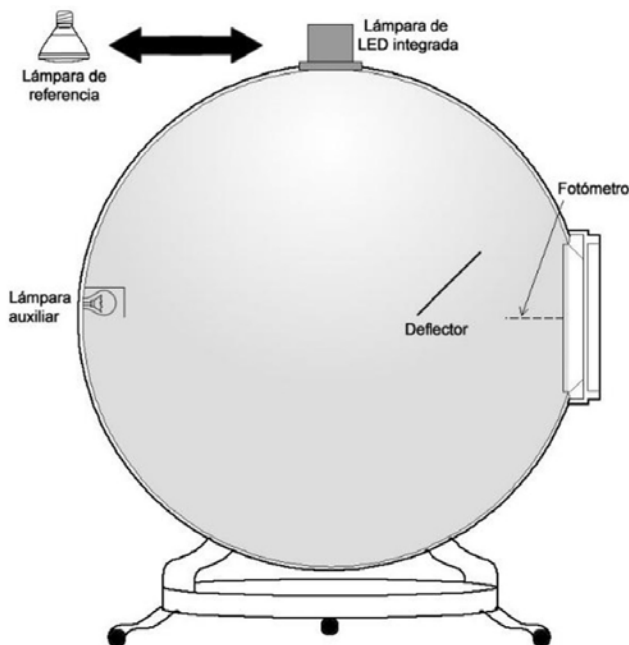
Figura K2 - Configuración de la esfera integradora 2\pi
