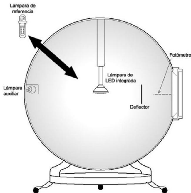
Figura K1 - Configuración de la esfera integradora 4\pi
