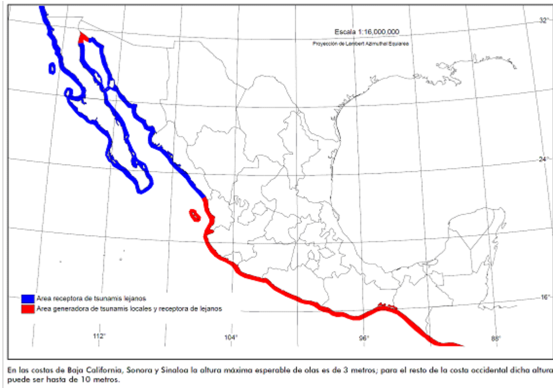
Figura 1 Mapa de peligros por tsunami (CENAPRED, 2001)
