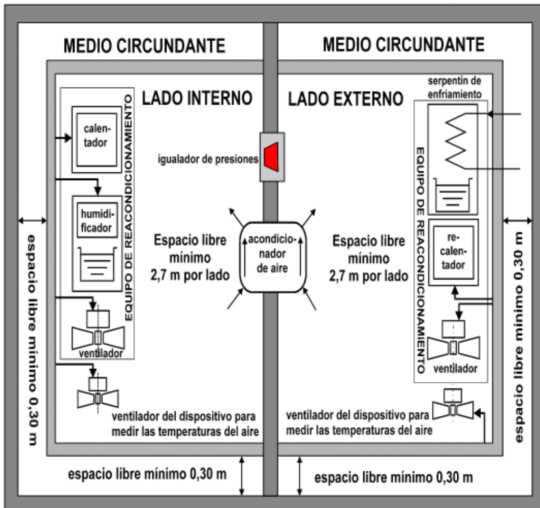
Figura 1. Calorímetro de cuarto tipo ambiente balanceado
