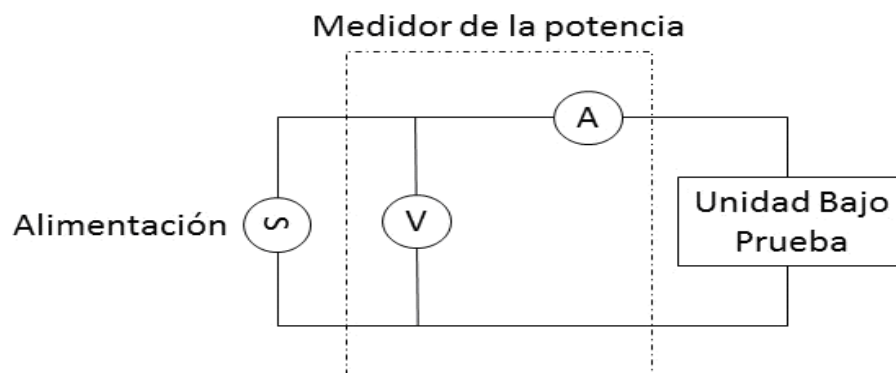
Figura 1. Arreglo de pruebas para las mediciones de potencia eléctrica en modo de espera
