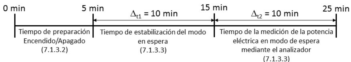
Figura 2. Diagrama secuencial para la obtención de la potencia eléctrica promedio.
