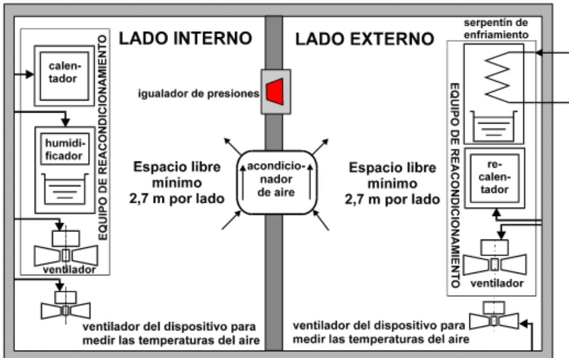
Figura 2. Calorímetro de cuarto tipo calibrado
