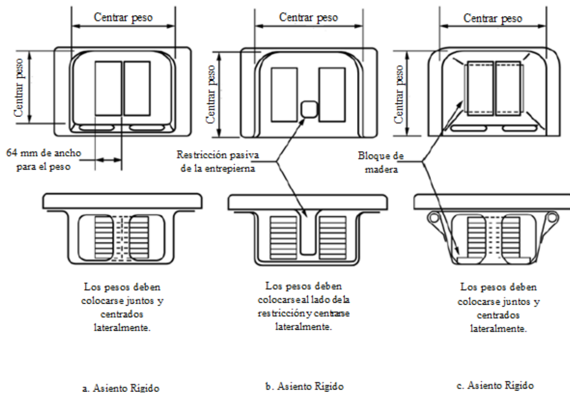
Figura 2 - Arreglo de pesos para prueba de estabilidad
