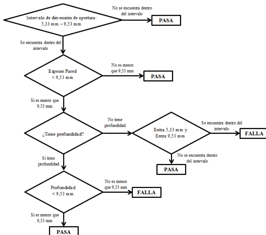
Figura 1 - Diagrama de Flujo para la determinación de orificios y aberturas.
