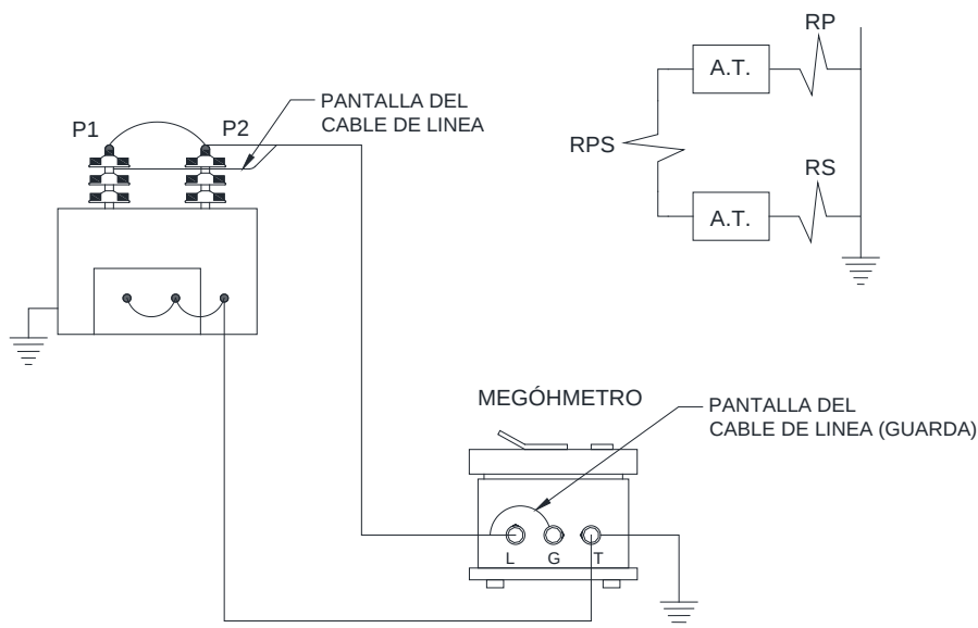
Figura 4. Diagrama de conexión para las pruebas de resistencia de aislamiento.
