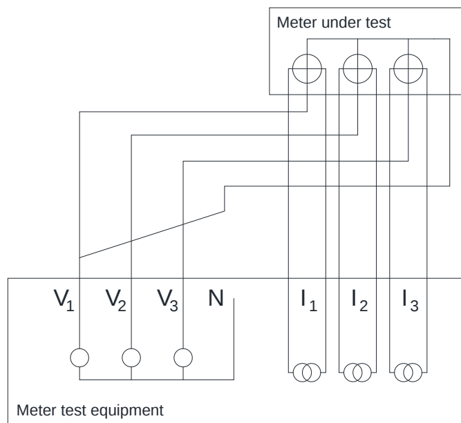
Figura 5. Esquema para la prueba de falla a tierra (en idioma inglés).
