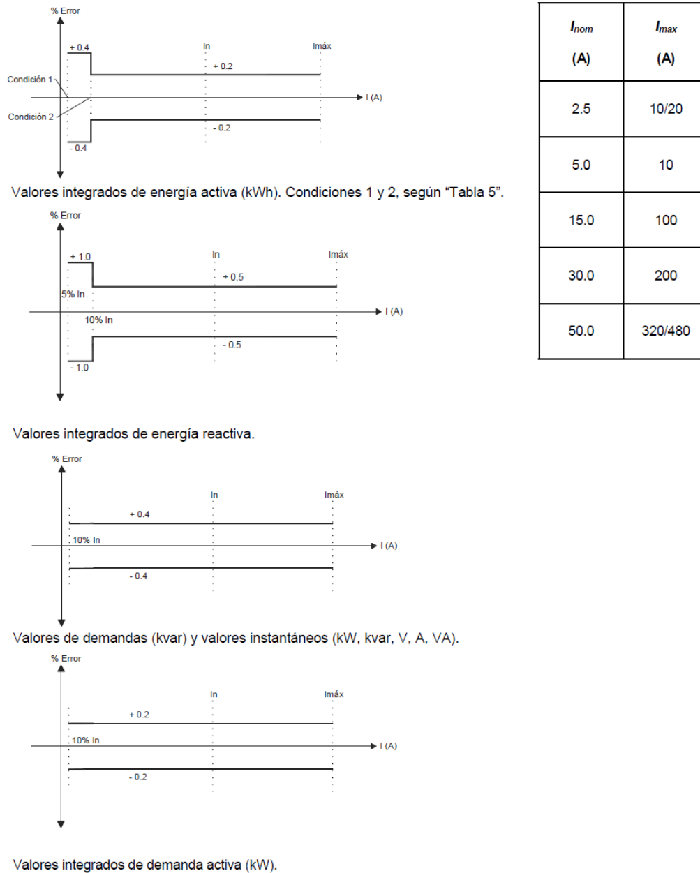
Figura 1. Gráficas de las envolventes del comportamiento de los medidores multifunción en condiciones de referencia V_{nom} , f.p. unitario, exactitud 0.2.
