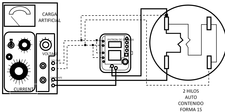
Figura 7. Diagrama de calibración con carga artificial sistema 1 fases 2 hilos con medidor autocontenido. inverso.
