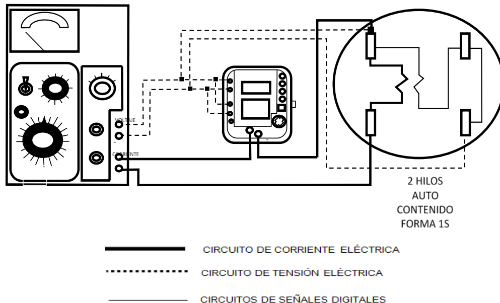
Figura 6. Diagrama de calibración con carga artificial sistema 1 fases 2 hilos con medidor autocontenido.
