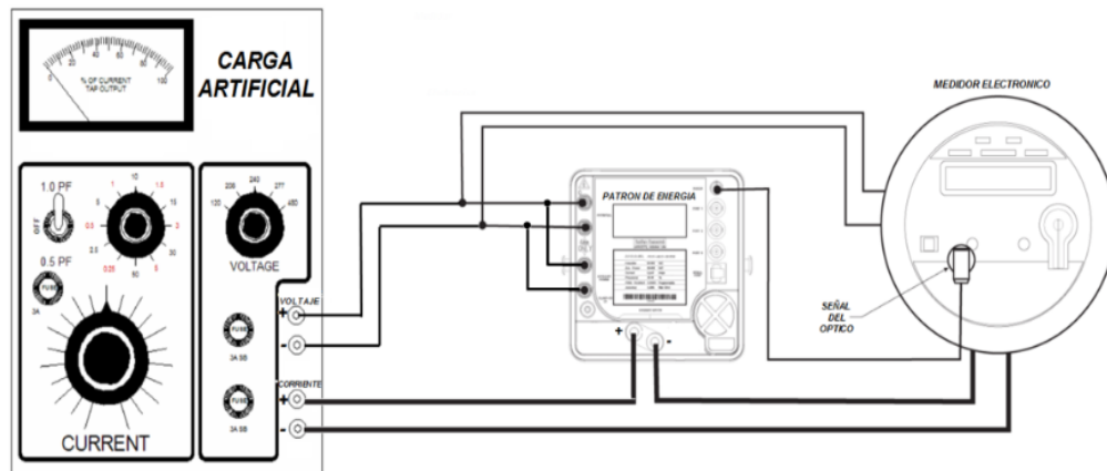
Figura 5. Diagrama de calibración con carga artificial sistema para medidor autocontenido.
