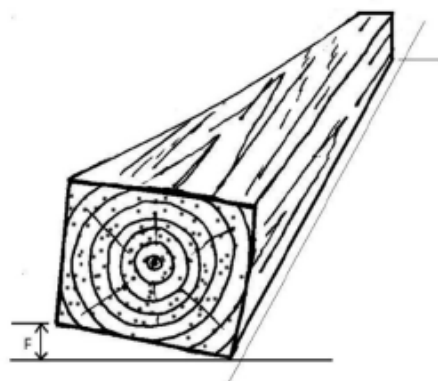
Figura 6. Torcedura
