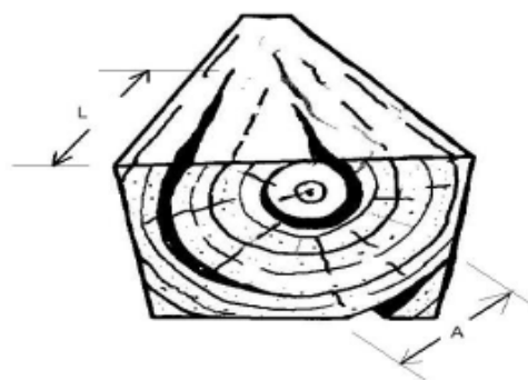
Figura 7. Acebolladuras
