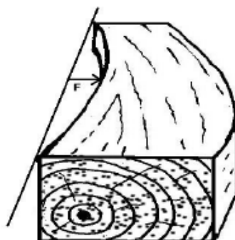
Figura 5. Encorvadura
