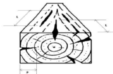
Figura 10. Grietas
