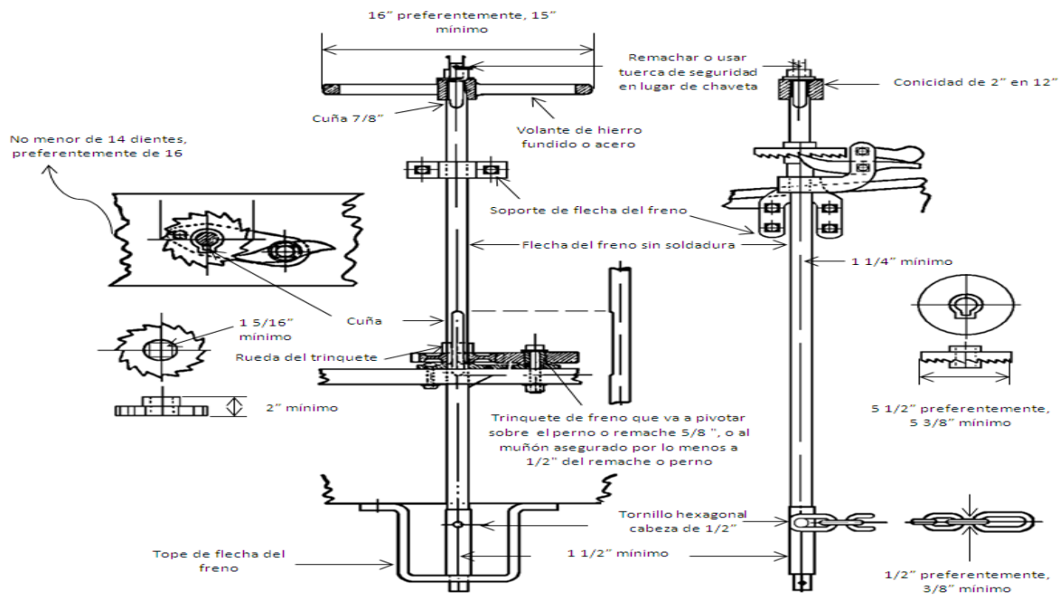
MECANISMO DEL FRENO DE MANO
