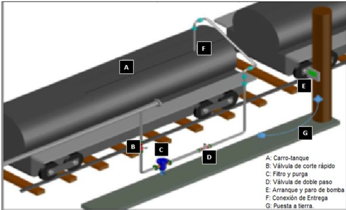
Figura 7. Sistema de Recepción de Carro-tanque
