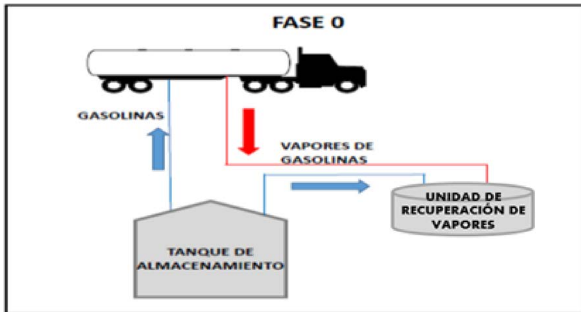
Figura 13. Fase 0 del Sistema de Recuperación de Vapores
