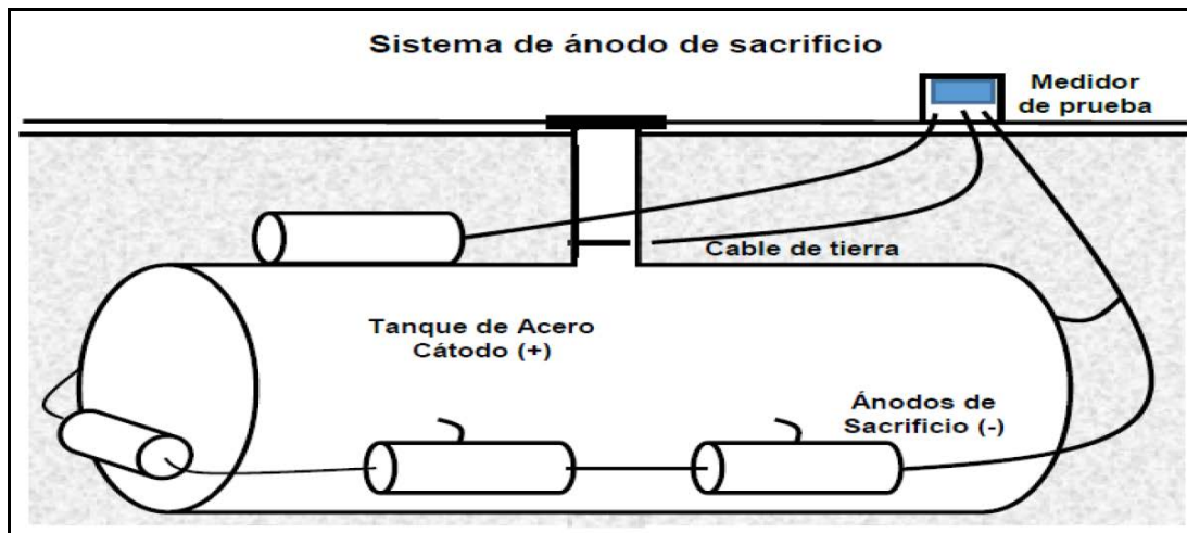
Figura 4. Sistema de protección catódica por ánodos de sacrificio
