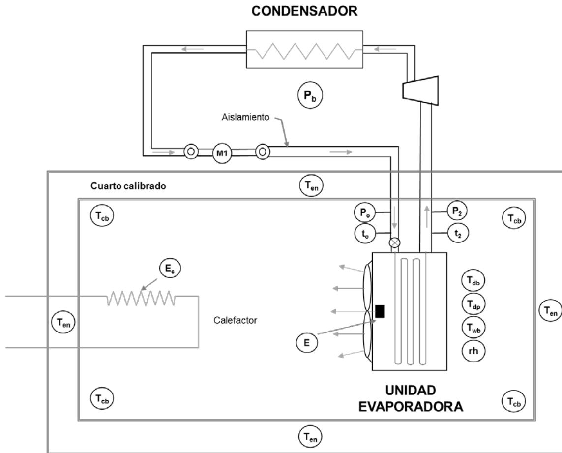
Figura 3.- Método cuarto calibrado
