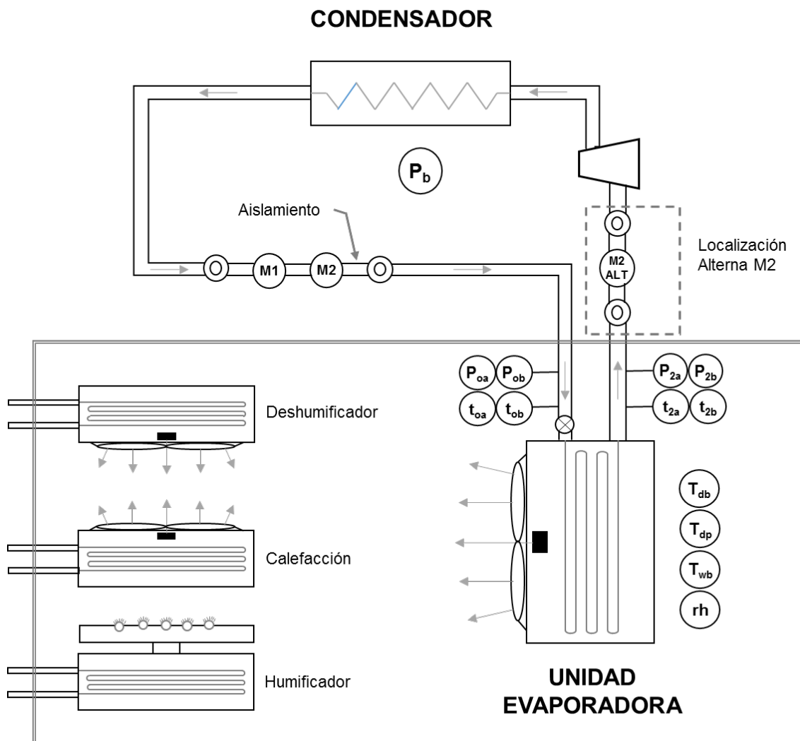
Figura 2.- Método doble instrumentación
