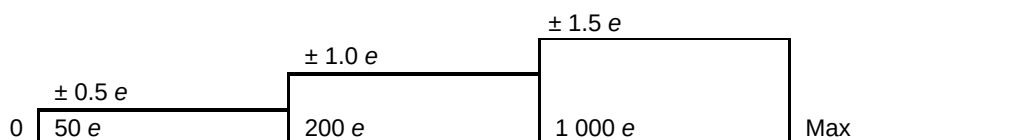
Figura 6-Errores máximos permitidos (emp) para la verificación inicial
