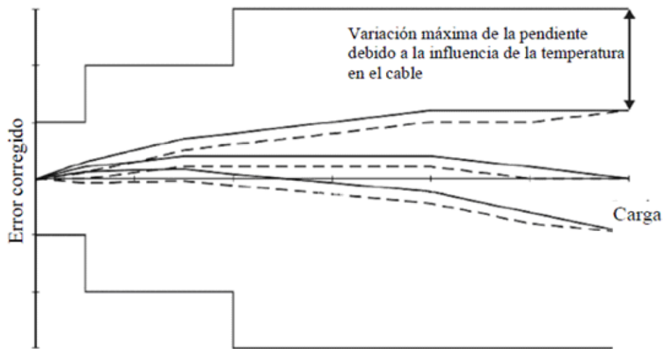
Figura C.1-Perfil de límites de variación del intervalo de pesada
