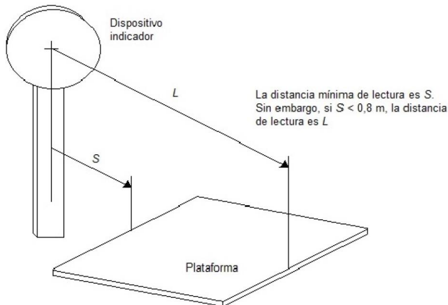
Figura 2-Representación para determinar la distancia mínima de lectura para el observador
