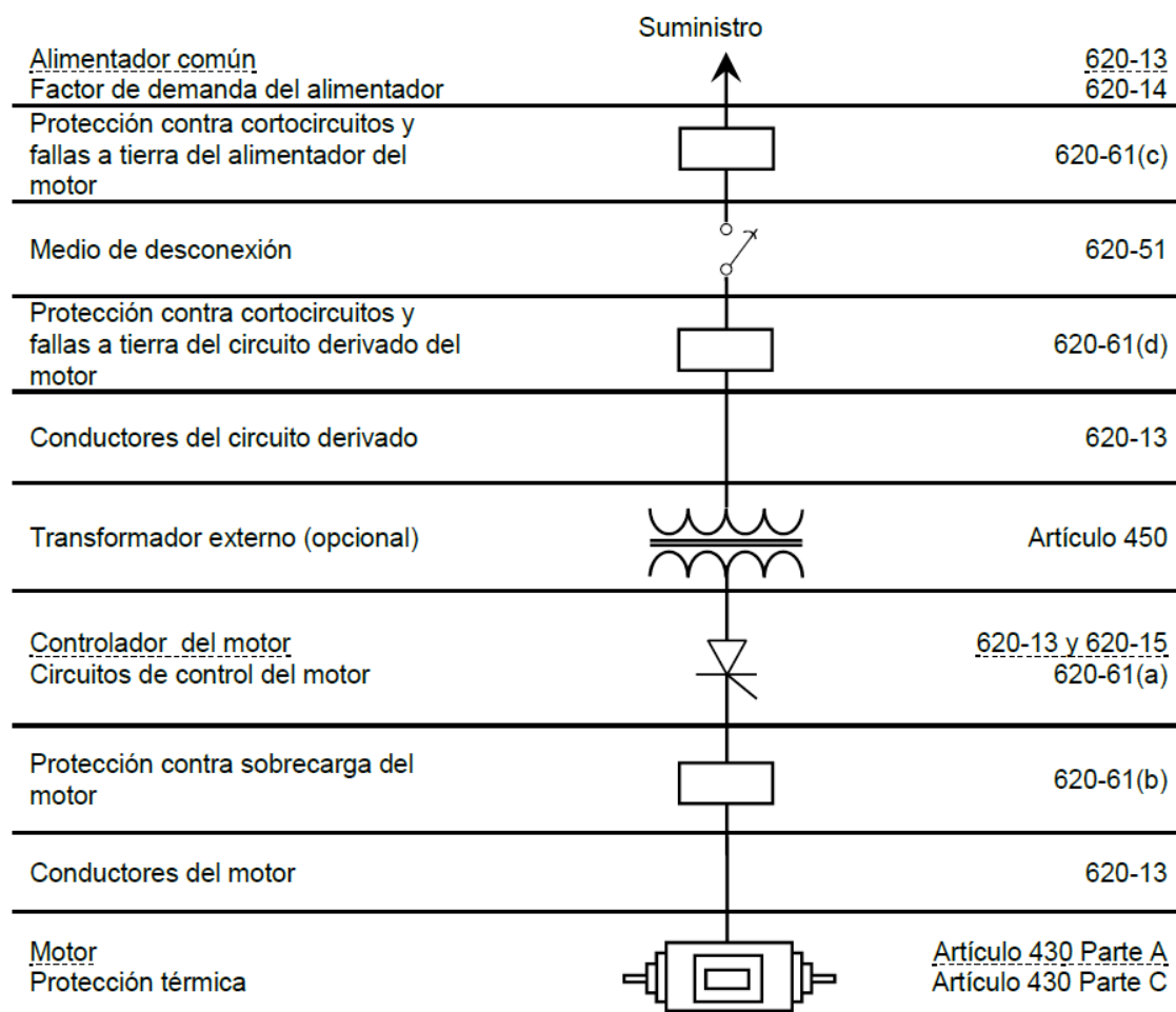
Figura 620-13.- Diagrama unifilar
