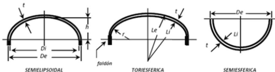
FIGURA A.1 FORMA DE LAS CABEZAS DE LOS RECIPIENTES
