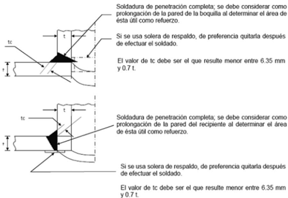
FIGURA A.2 ALGUNOS TIPOS PERMITIDOS DE BOQUILLAS SIN ESFUERZO
