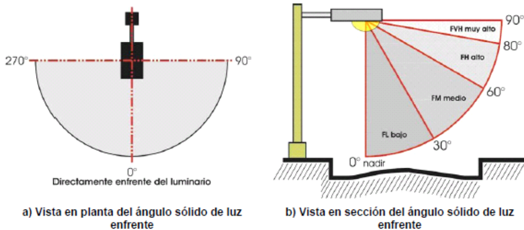
Figura D4. Ángulos sólidos secundarios verticales para luz enfrente o lado calle
