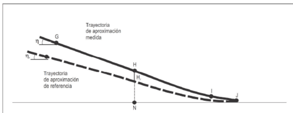
Figura A1-8. Comparación de los perfiles de aproximación medidos y corregidos.
