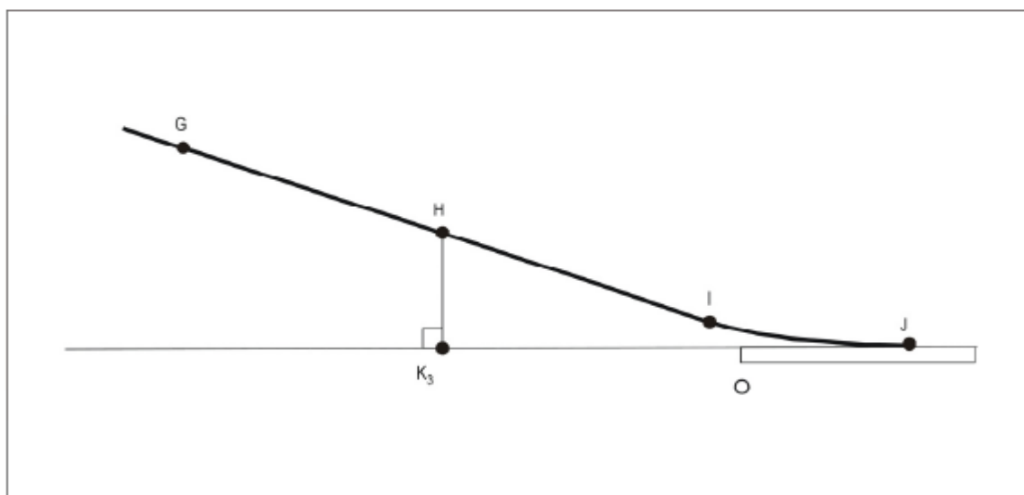
Figura A2-6. Características del perfil de aproximación de referencia para aeronaves de ala fija.
