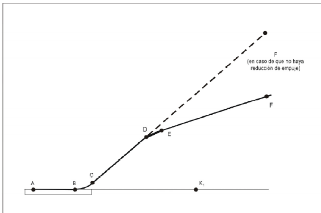
Figura A2-5. Características del perfil de sobrevuelo de referencia para aeronaves de ala fija.
