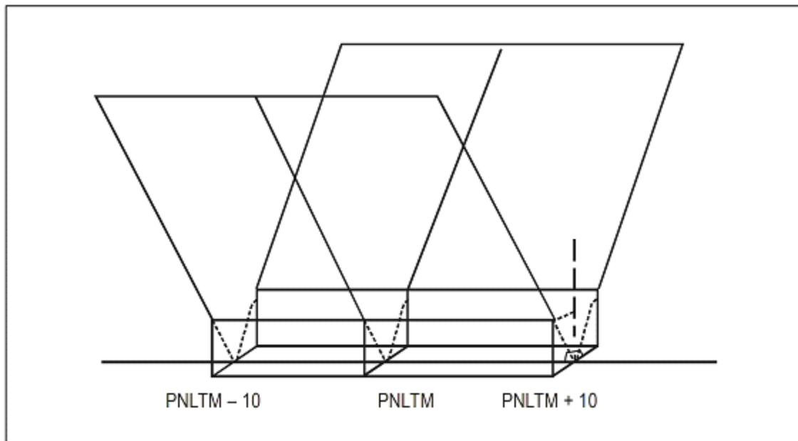
Fig. 11-1 Tolerancia de desviación lateral de los helicópteros.
