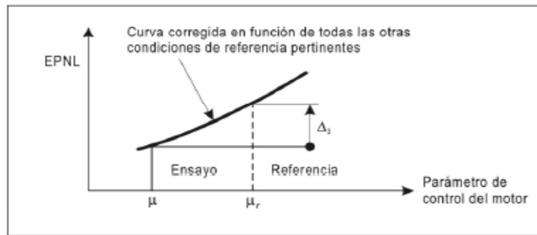
Figura A2-12. Ajuste del ruido en la fuente.
