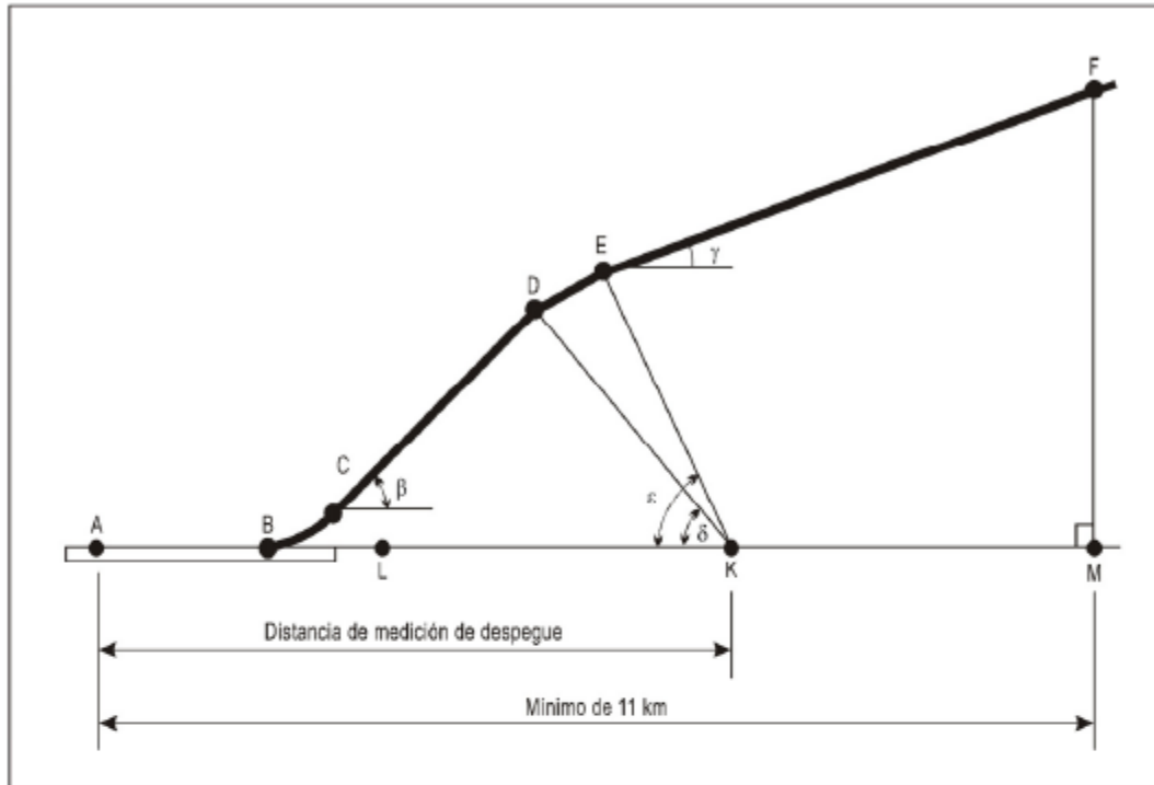
Figura A1-4. Perfil de despegue medido.
