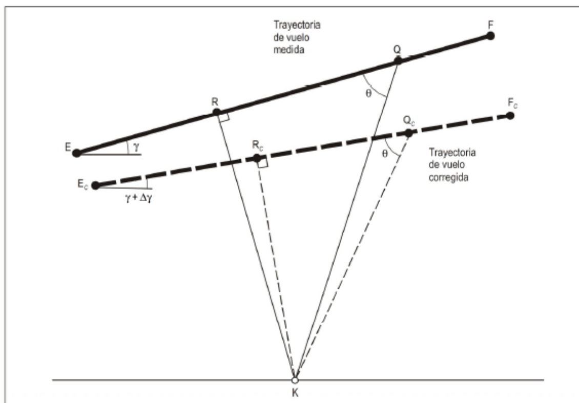
Figura 1-6. Características del perfil de despegue que influyen en el nivel acústico.
