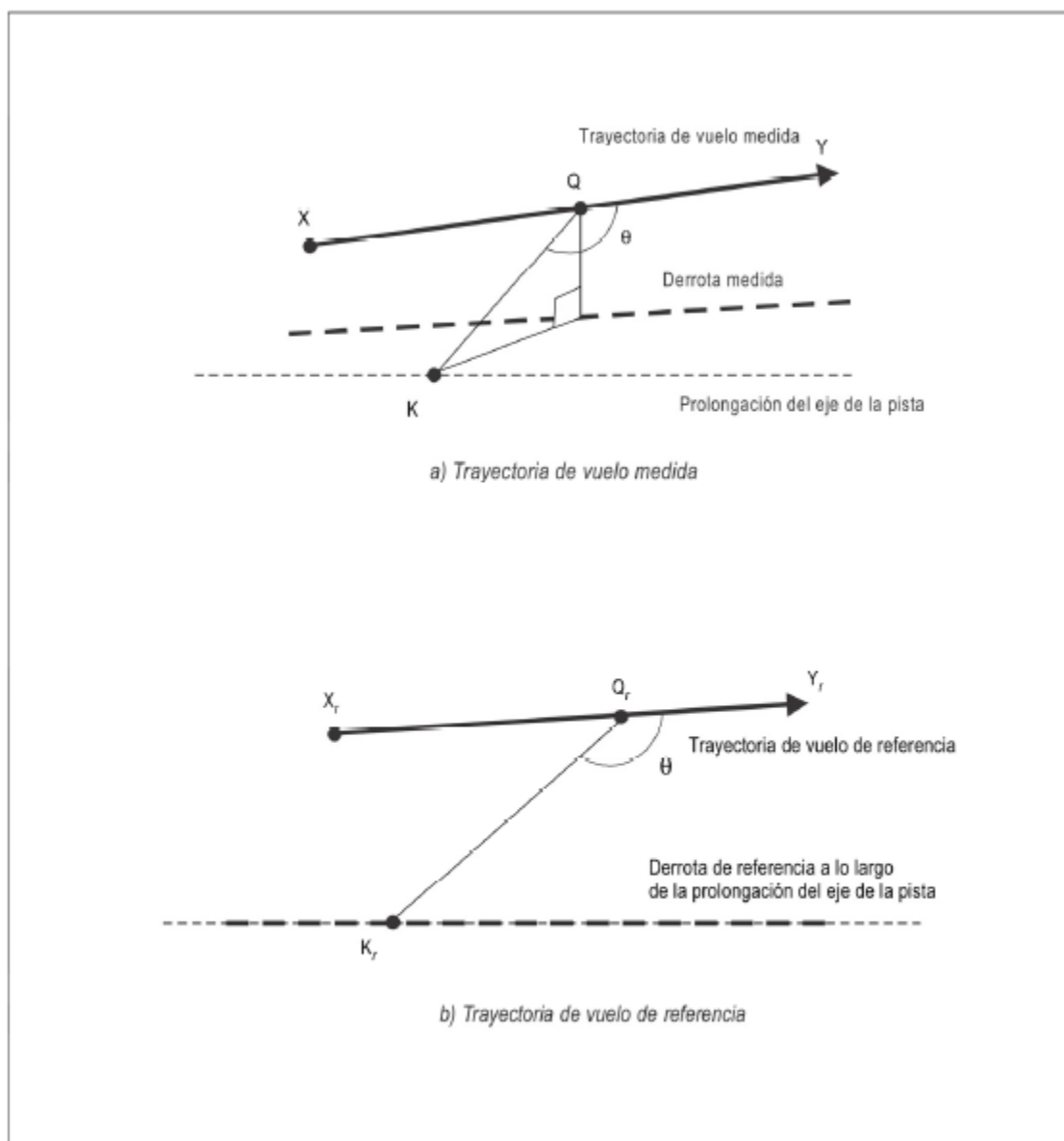
Figura A2-10. Características de perfil que influyen en el nivel acústico para micrófonos emplazados debajo de la trayectoria de vuelo.
