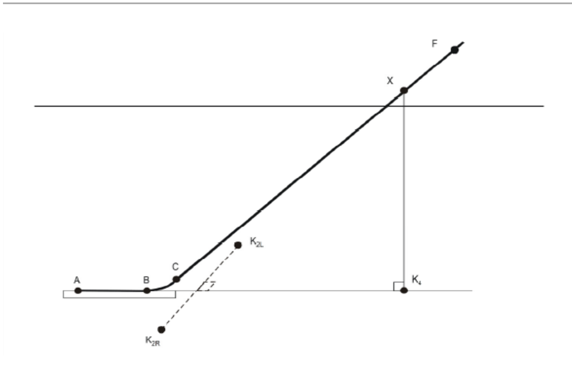
Figura A2-4. Características del perfil de ruido lateral con plena potencia de referencia para aviones.
