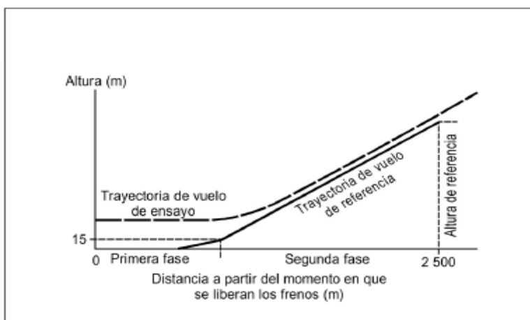
Figura A6-1. Perfiles de ensayo y de referencia típicos.
