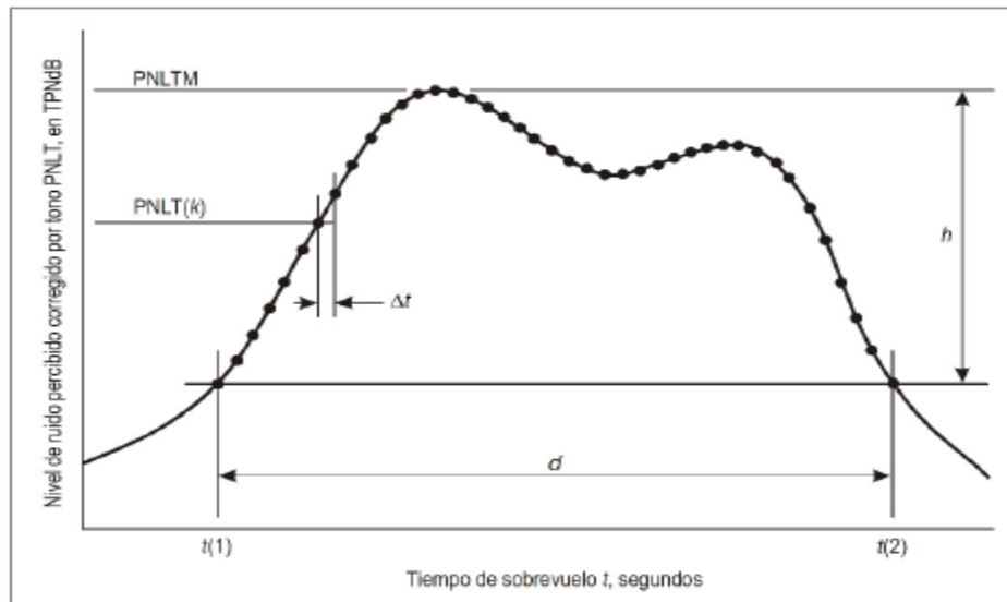
Figura A1-2. Ejemplo del nivel de ruido percibido corregido por tono en función del tiempo de sobrevuelo de la aeronave.
