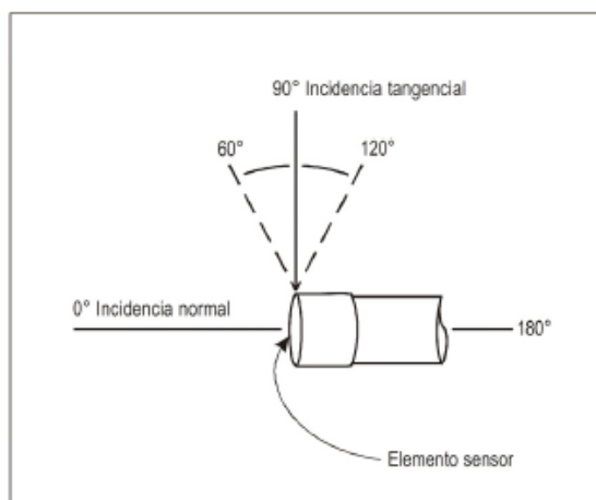
Figura A2-1. Ilustración de los ángulos de incidencia sonora en micrófono.
