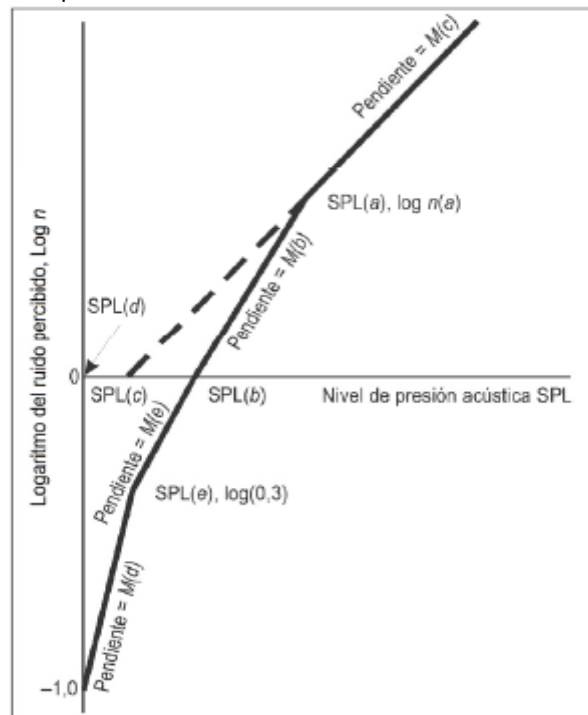
Figura A2-3. Ejemplo del nivel de ruido percibido corregido por tono, en función del tiempo de sobrevuelo del avión
