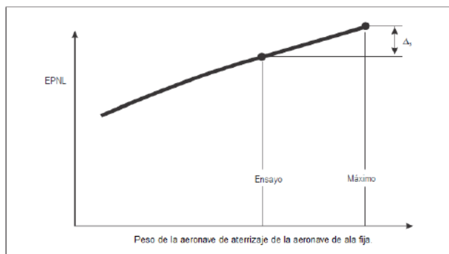
Fig. A1-11. Corrección del peso de aproximación correspondiente al EPNL.
