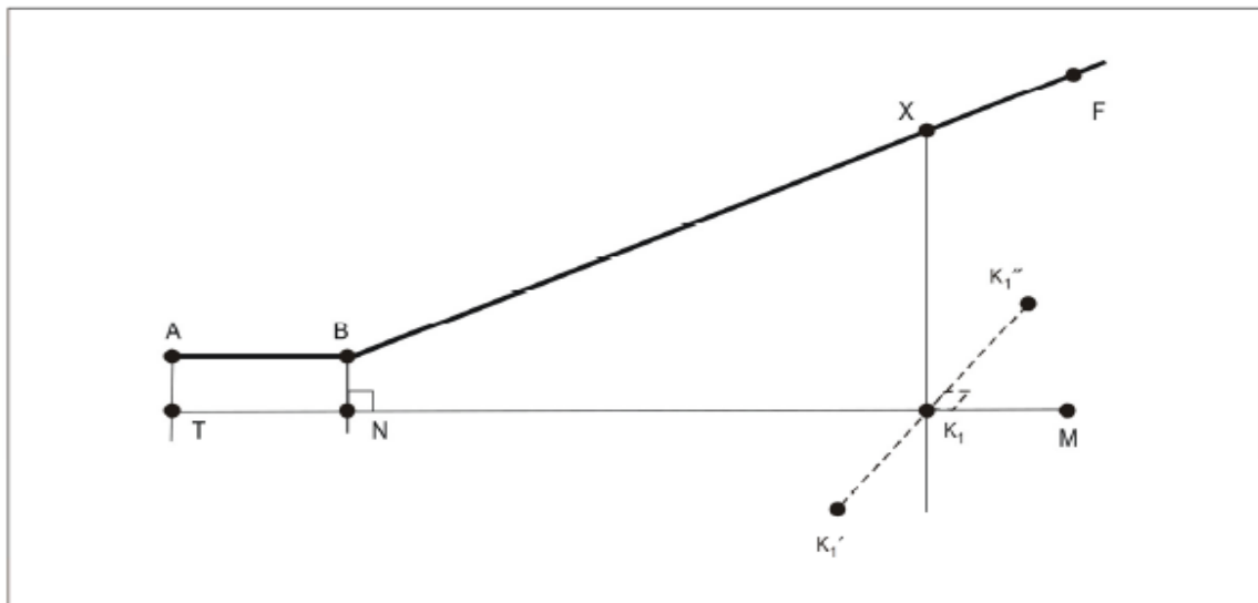
Figura A2-7. Características del perfil de despegue de referencia para helicópteros.
