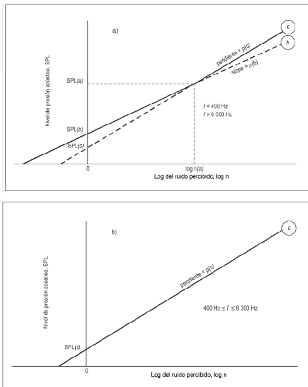
Fig. A1-3. Nivel de presión acústica en función del ruido percibido.
