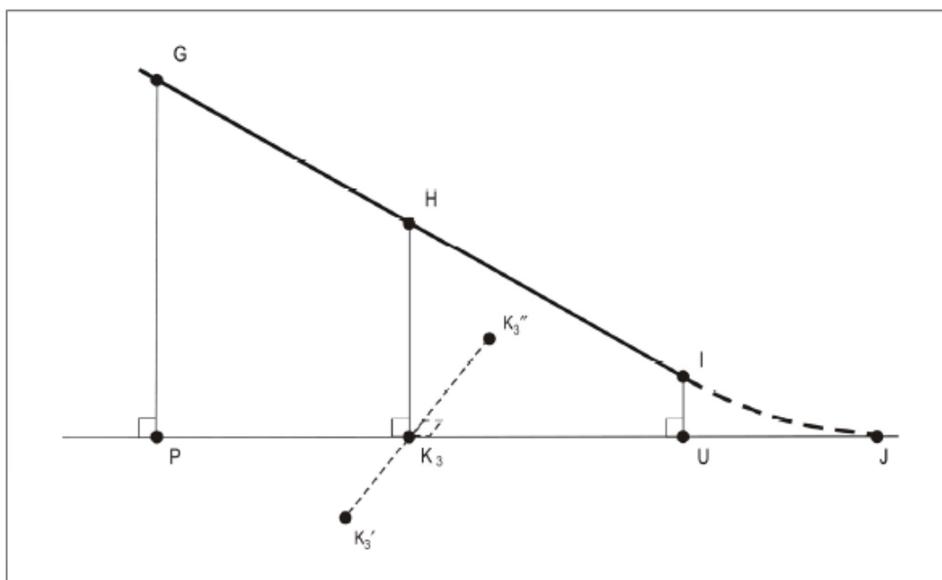
Figura A2-9. Características del perfil de aproximación de referencia para helicópteros.
