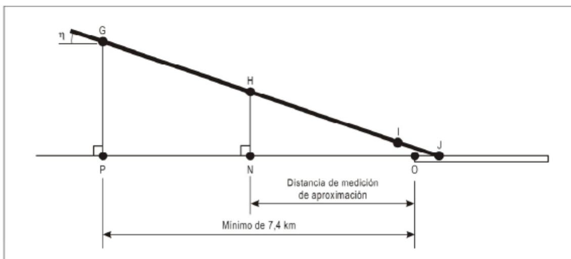
Figura A1-7. Perfil de aproximación medido.
