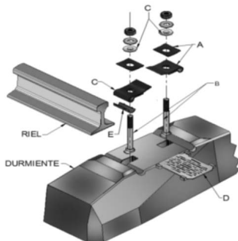
Figura 5. Sistema de fijación en vía elástica
