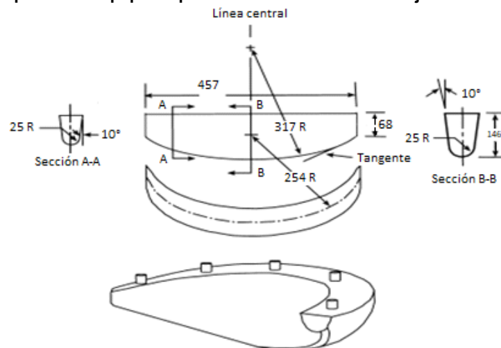
Figura 1-Eschema del equipo de prueba de resistencia de la ceja al desmontaje del rin.
