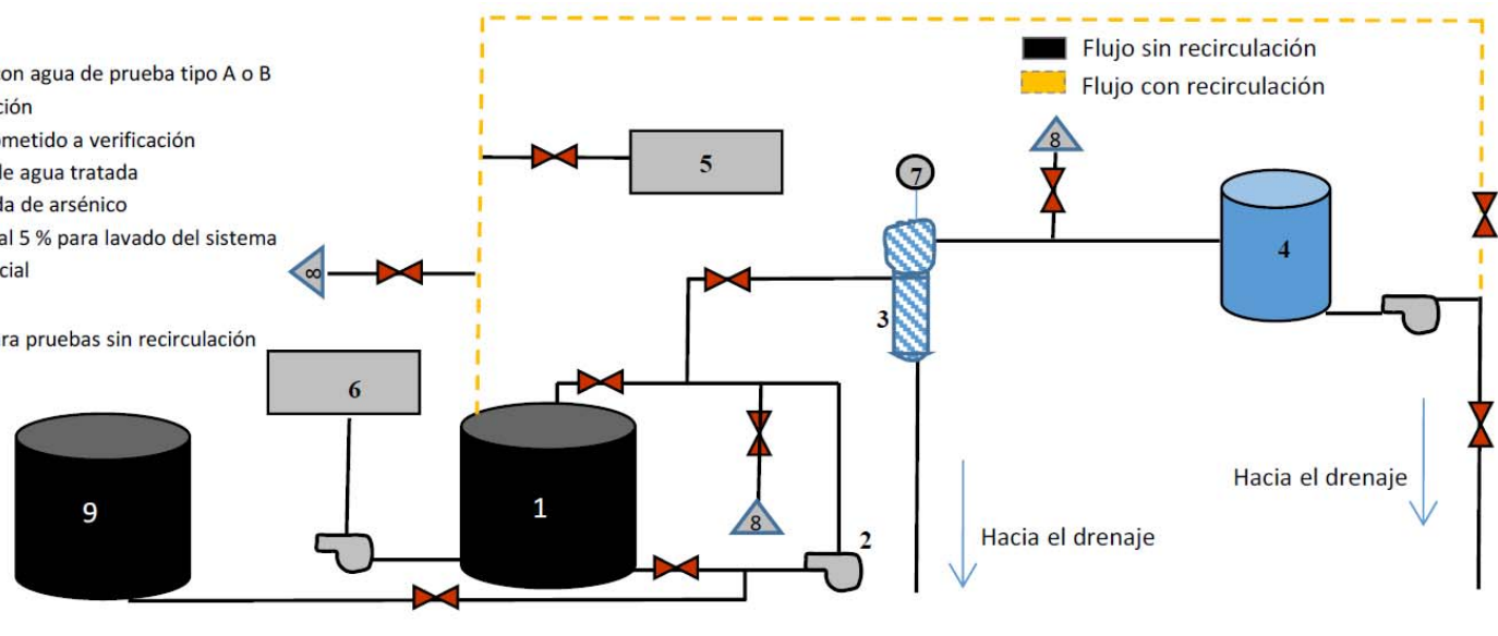
Figura G.1. Montaje para la verificación de equipos en la remoción de Arsénico en Agua para uso y consumo humano.
