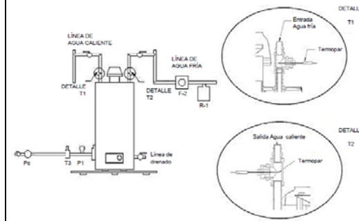
FIGURA 2-Calentador de rápida recuperación (ilustrativa no limitativa)
