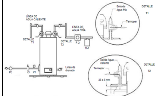
FIGURA 1-Calentador de almacenamiento (ilustrativa no limitativa)
