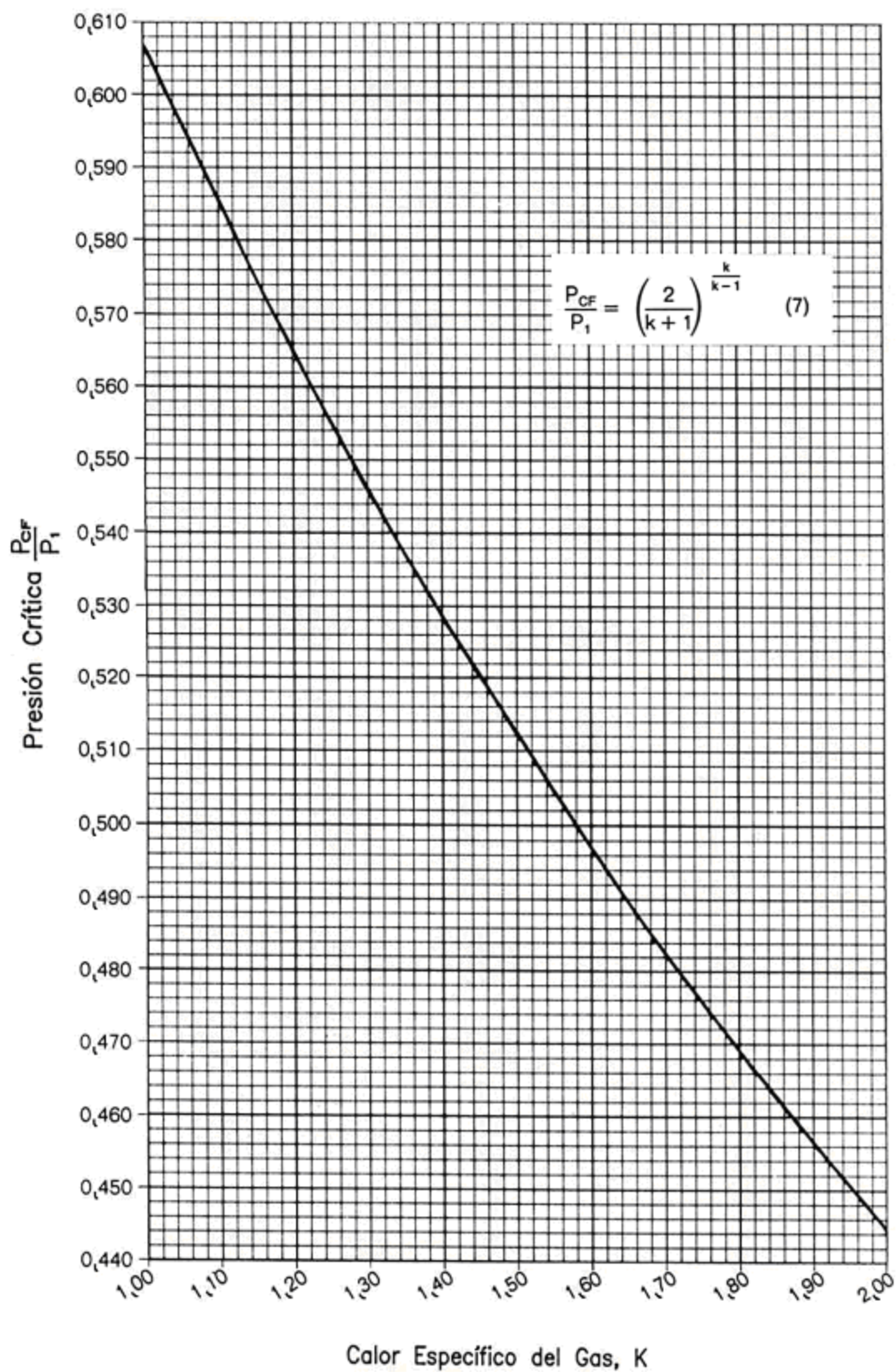
Figura ilustrativa C2 - Curva para determinar el valor de la presión crítica P_{cf}/P_1
