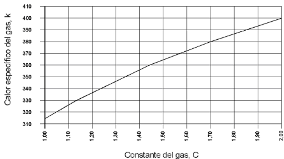
Figura ilustrativa C1 - Curva para determinar la constante C del gas y el valor del calor específico del gas
