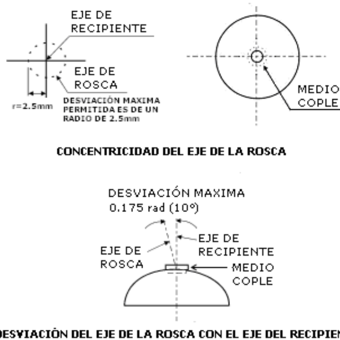
Figura 15 - Concentricidad y desviación del medio cople con el recipiente
