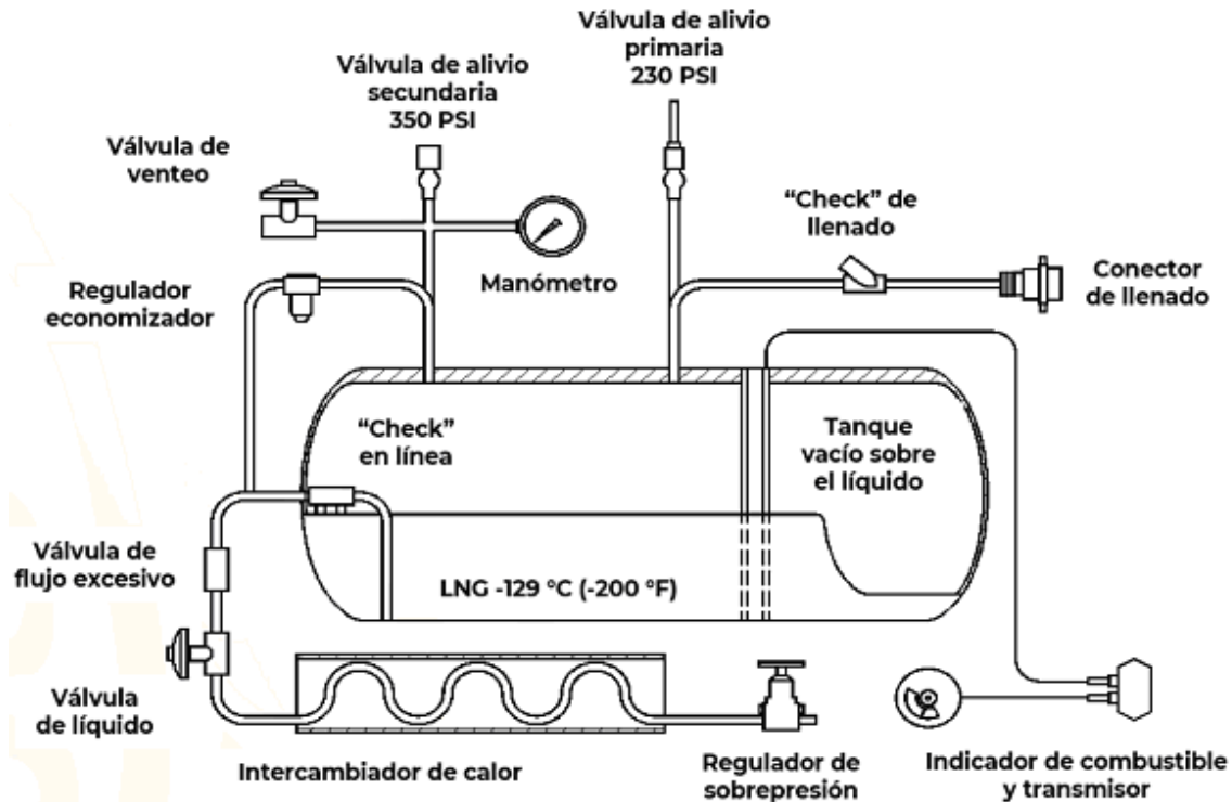
Diagrama 2 - Componentes de Gas Natural Licuado (ilustrativo no limitativo)
