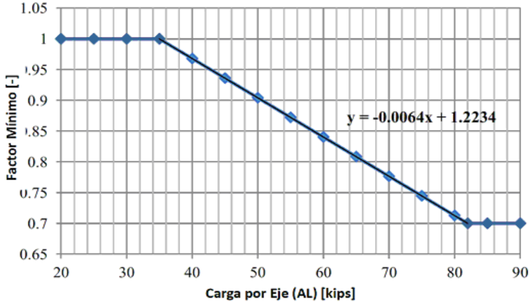
Figura 5. Límite para Factores de Tonelaje y Velocidad
