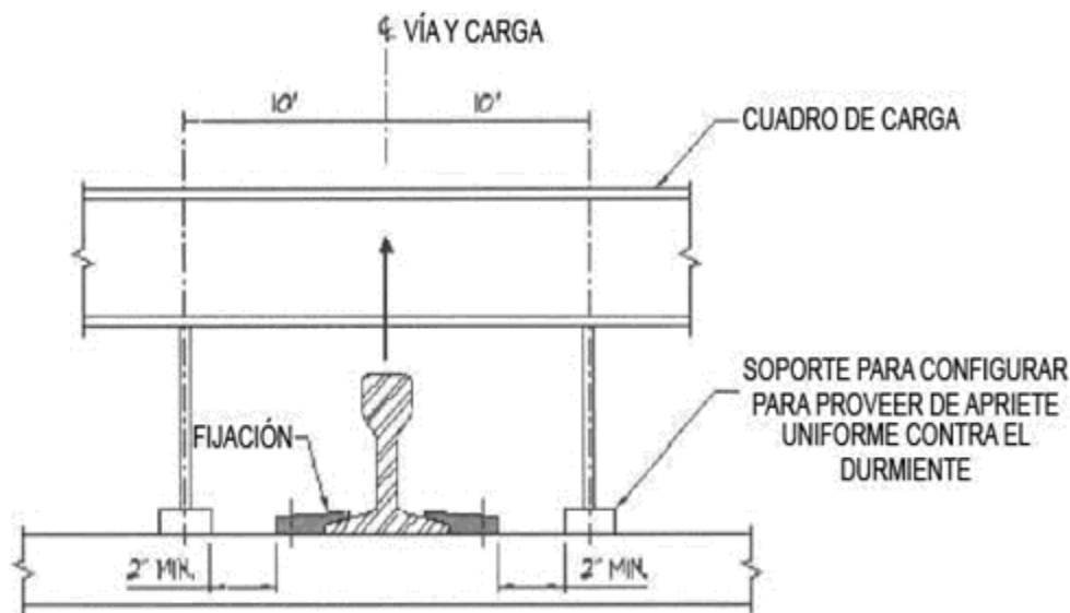
Figura 14. Prueba de extracción de Fijación
