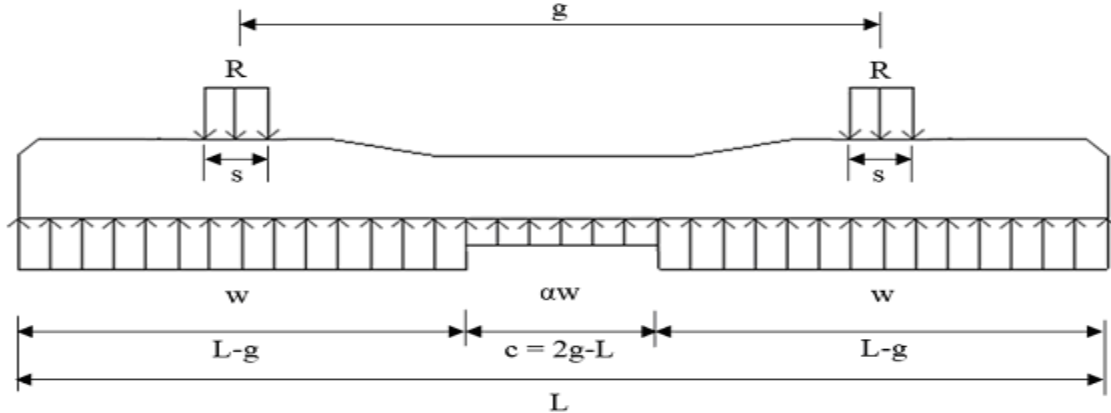
Figura 2. Condiciones de Carga y de Apoyo Supuestas para la Determinación de Momentos Flexionantes de Diseño
