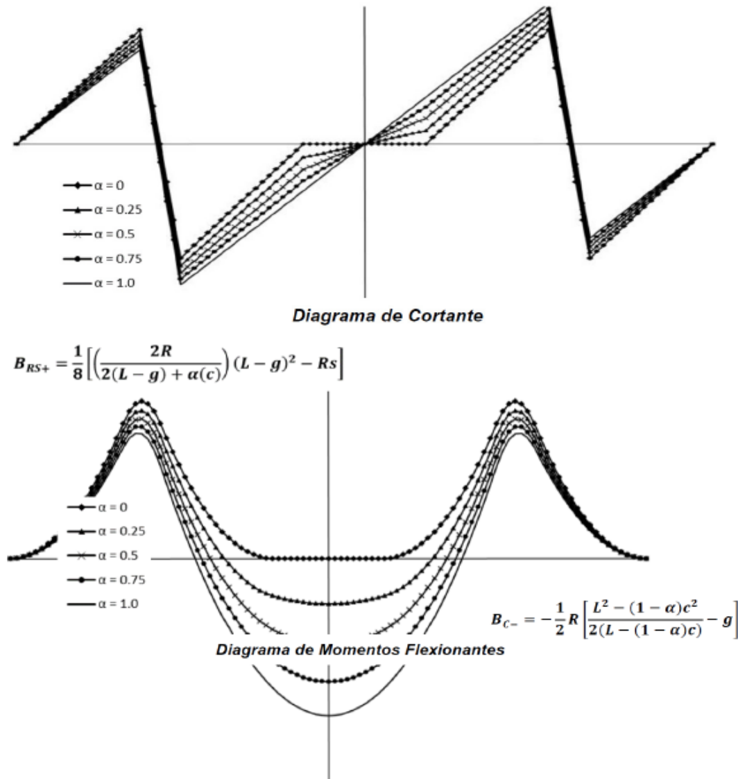
Figura 4. Suposiciones de Carga y Condiciones de Soporte, Diagrama de Cortante y Diagrama de Momento Flexionantes para la Determinación de Momentos Flexionantes de Diseño
