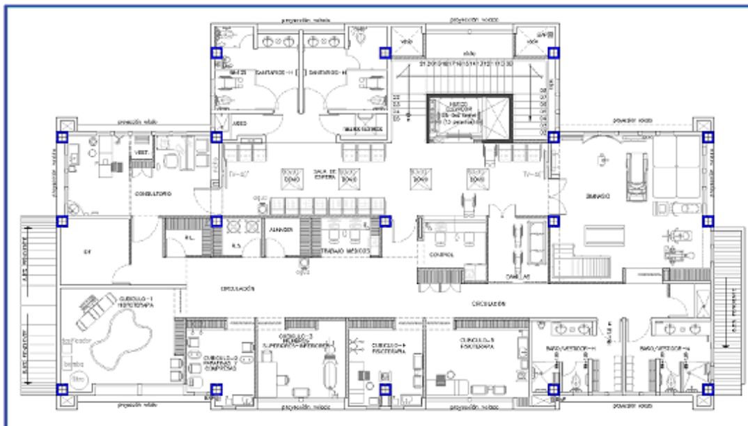
2. PLANTA ALTA. Edificio Cámara Hiperbárica
