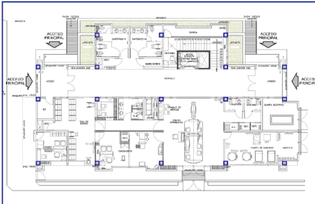
1. PLANTA BAJA. Edificio Cámara Hiperbárica
