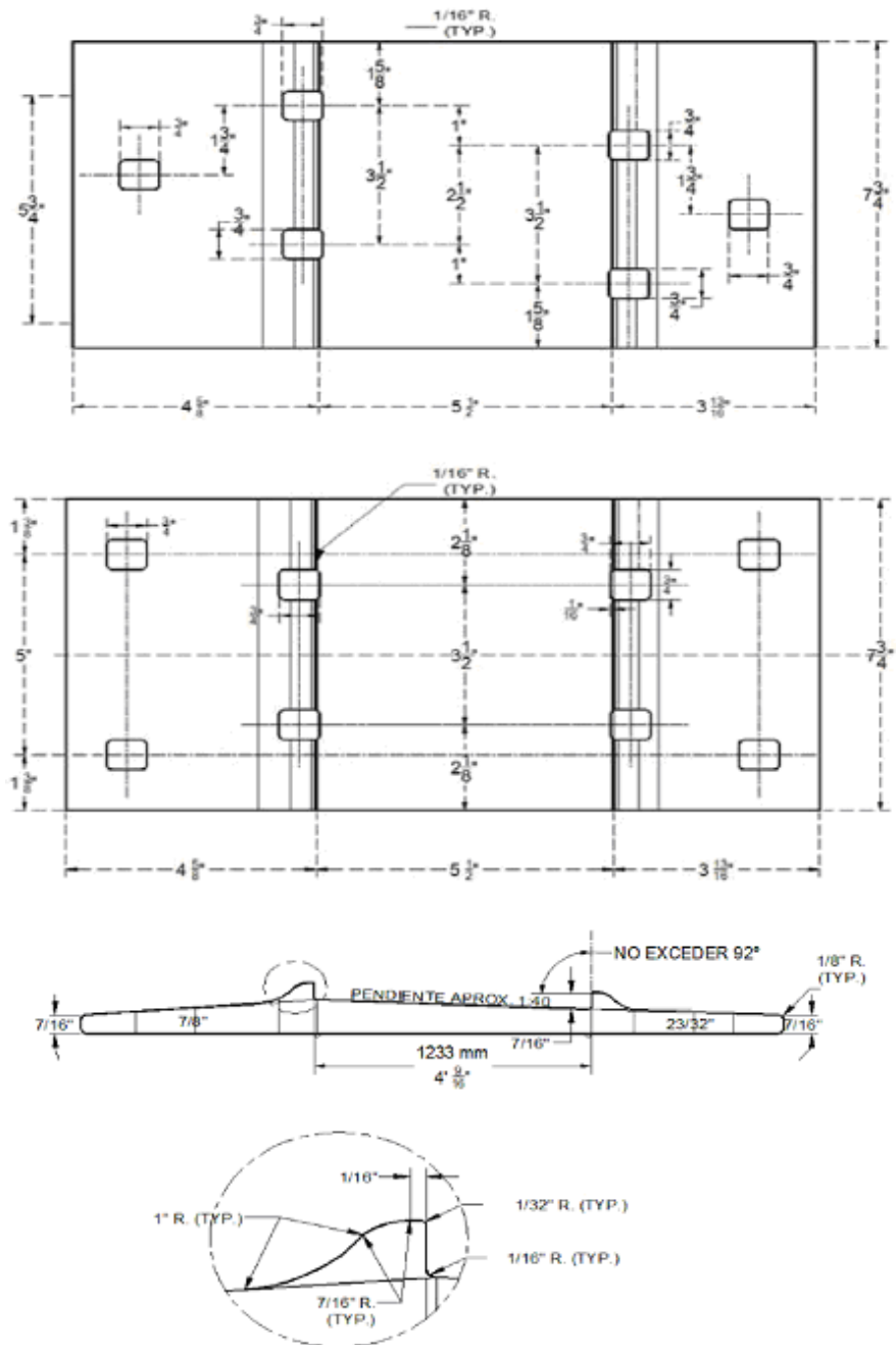
Figura 6-Placas de asiento
