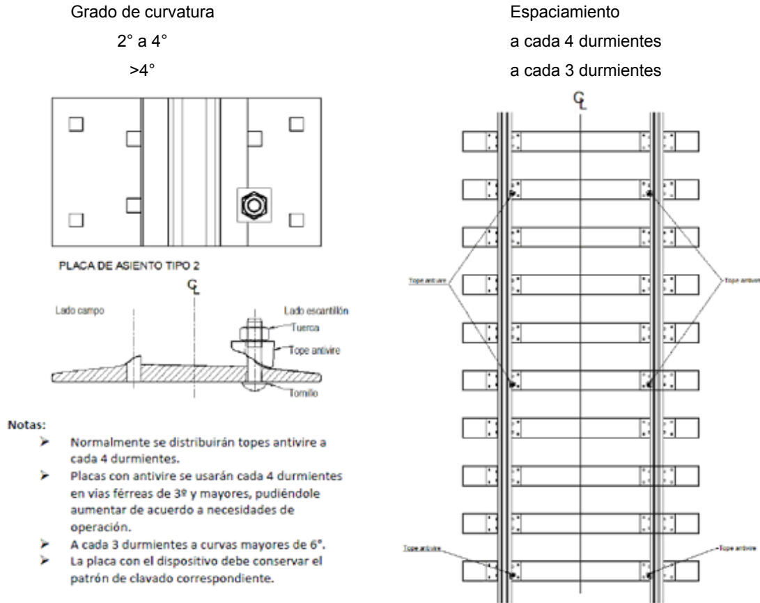
Figura 8-Dispositivos antivire
