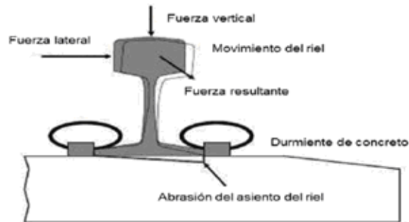
Figura 16-Desgaste de durmiente.
