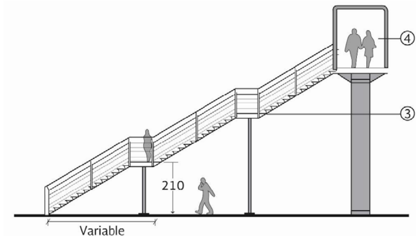
39 ALZADO DE PUENTE PEATONAL
