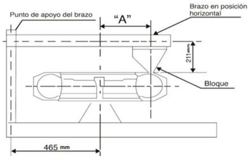
Figura 1-Eschema del equipo de prueba de resistencia de la ceja al desmontaje del rin
