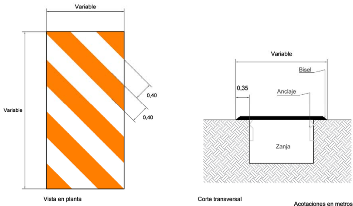
FIGURA 21.- Cubrezanjas
