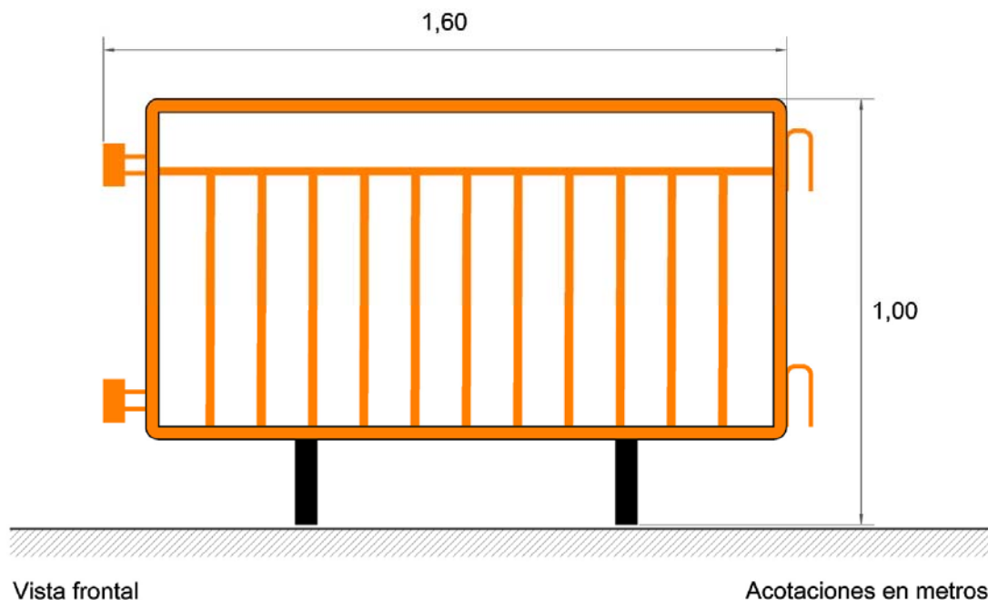
FIGURA 19.- Barrera de protección peatonal
