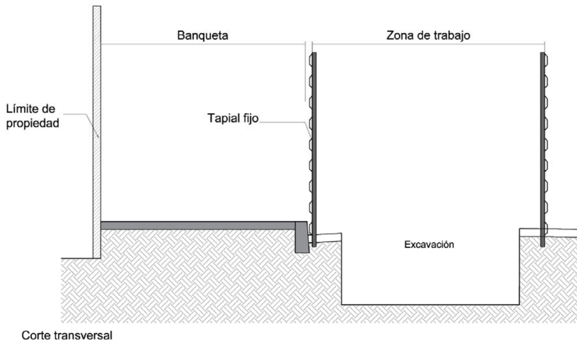
FIGURA 16.- Tapial fijo
