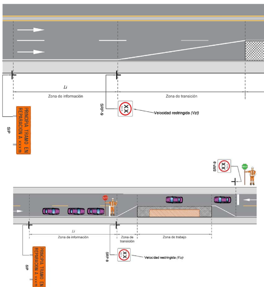
FIGURA 23.- Señales verticales que indican el principio y fin de la zona de información (Li)
