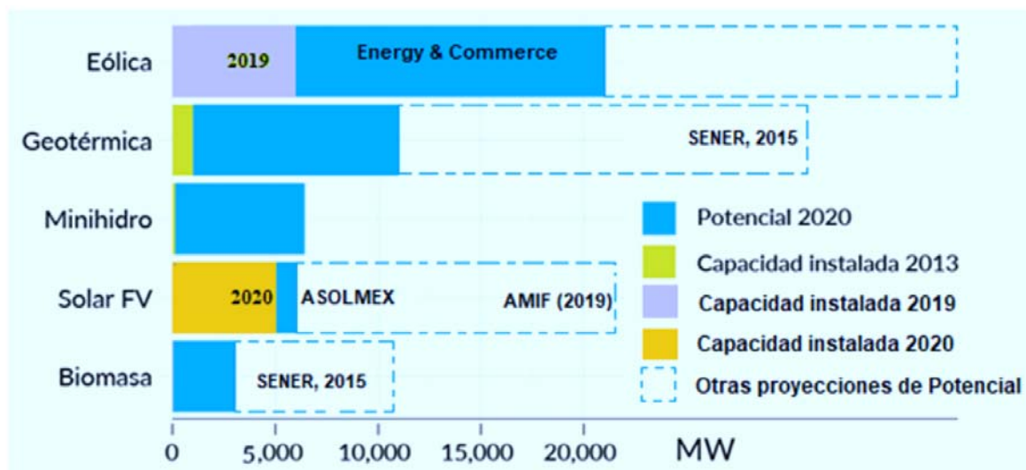
Figura 6. Situación actual de uso y potencial de las energías renovables en México (Escamilla, 2021).
