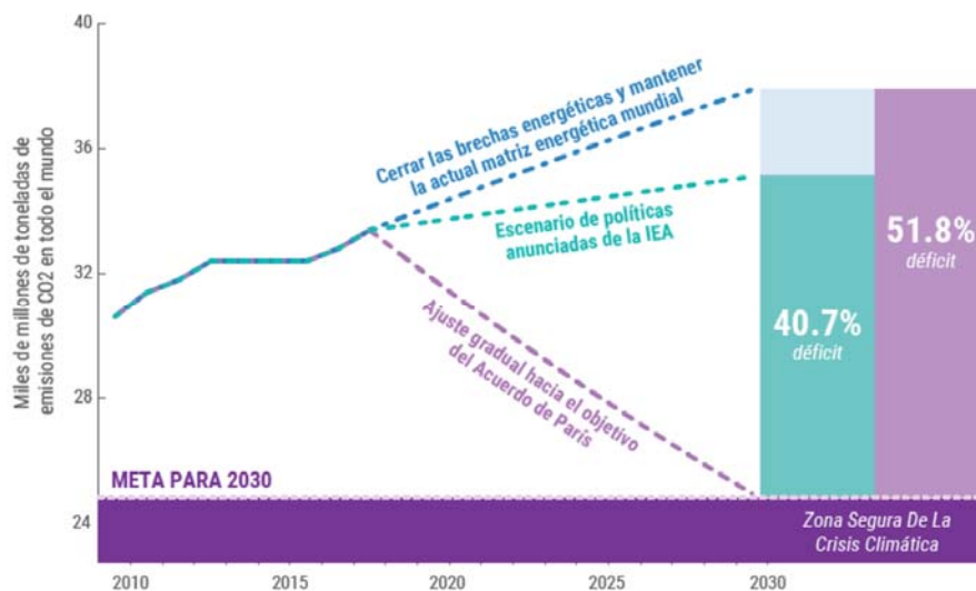
Figura 5. Diferentes escenarios de evolución de las emisiones de CO 2 mundial. Fuente (ONU, 2020)
