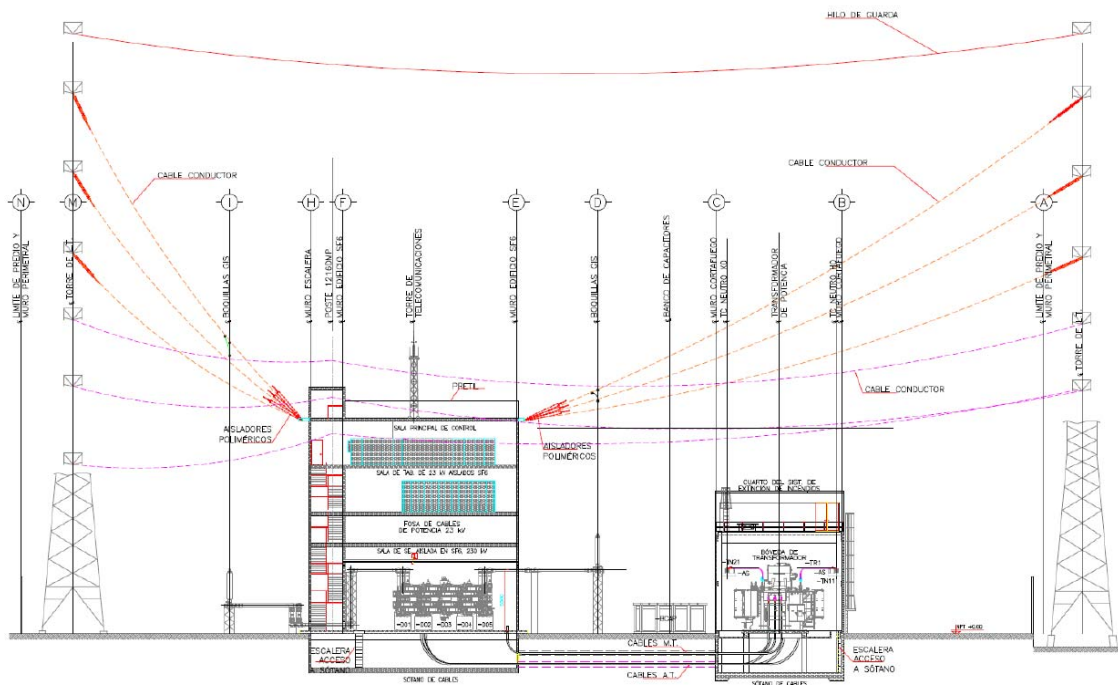
Figura 32 - Punto de conexión o interconexión aérea - con Edificio SF_6
