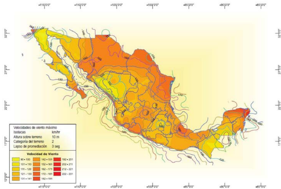
Figura 47 - Mapa de Isótopas para periodo de retorno de 50 años
