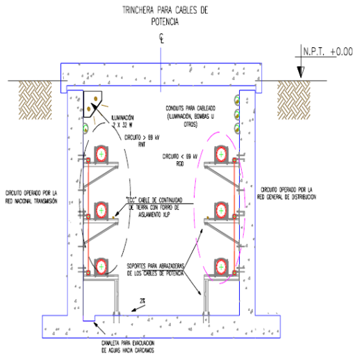
Doble circuito
