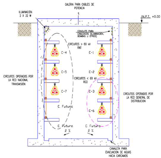
Múltiples circuitos
