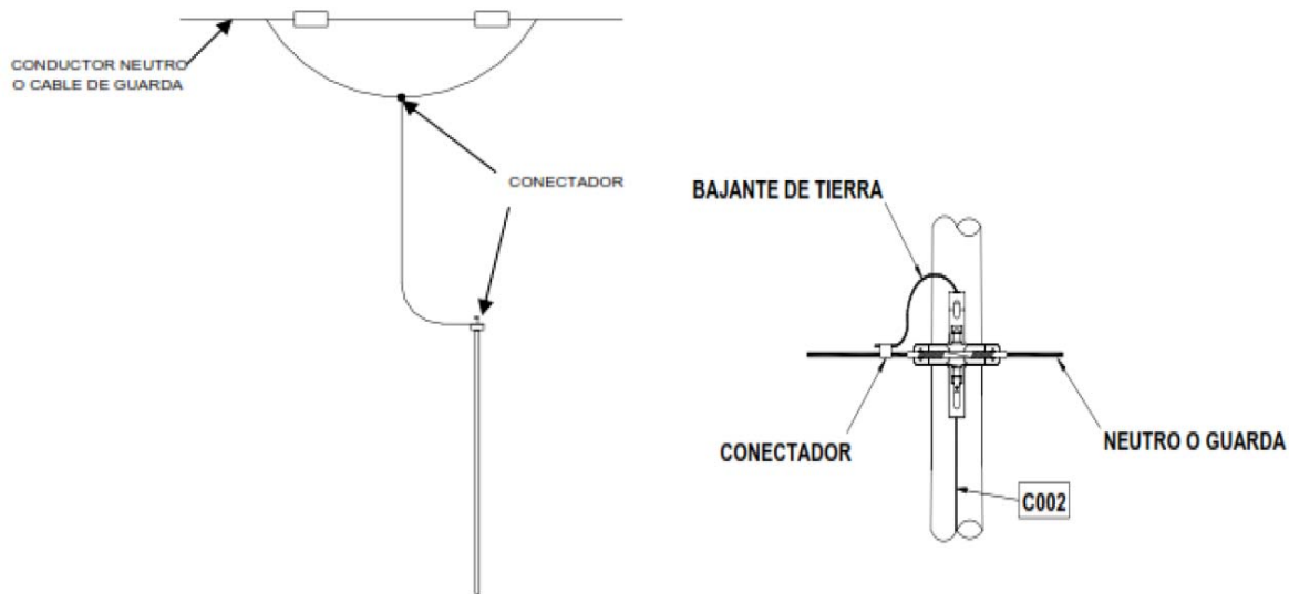
Figura 16 - Conexión de cable de neutro corrido con cable de guarda.
