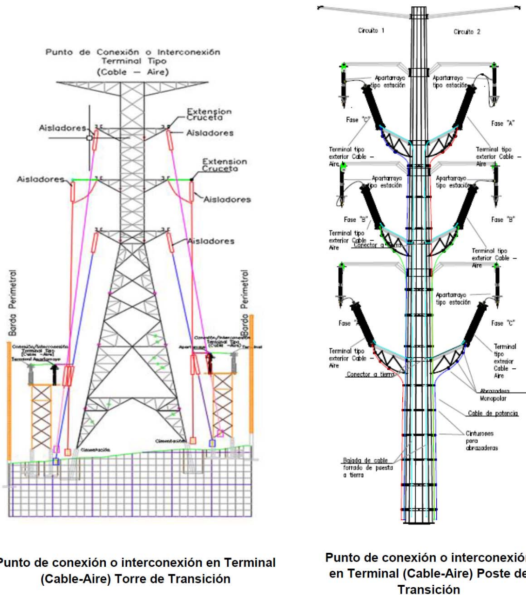
Figura 35 - Punto de conexión o interconexión subterránea - Punto de Interconexión en Transición Aéreo - Subterráneo
