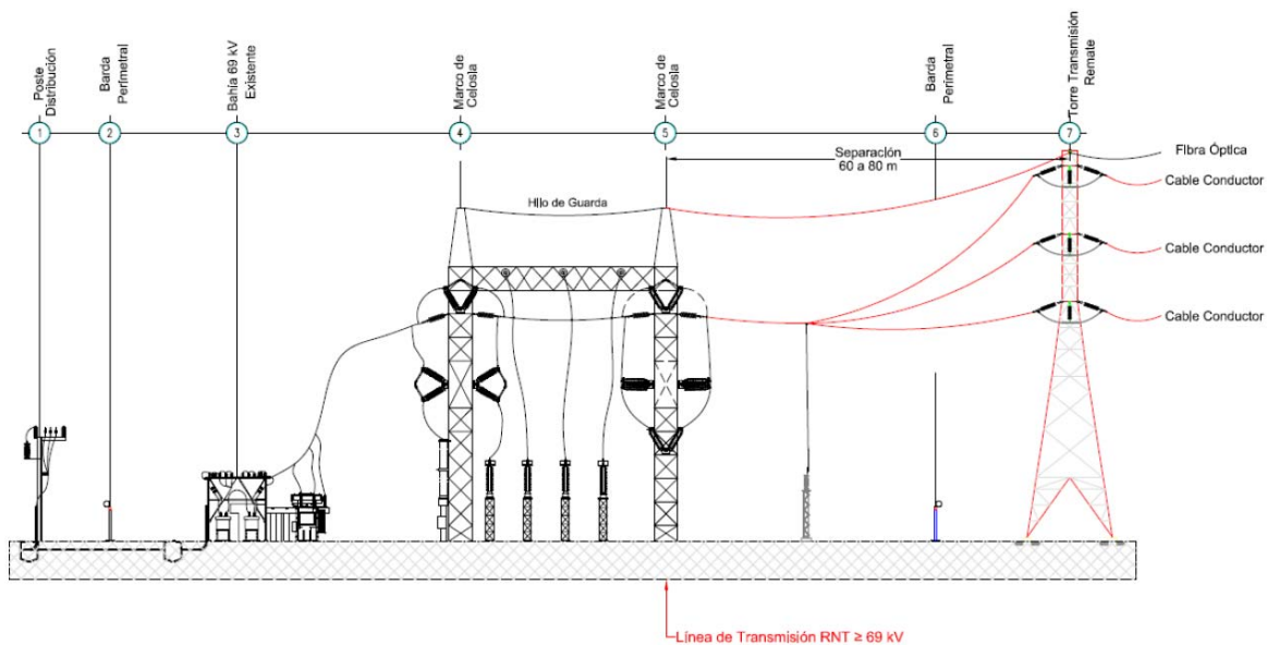
Figura 31 - Punto de conexión o interconexión aérea - Arreglo de Salida de Línea de Subestación de Distribución
