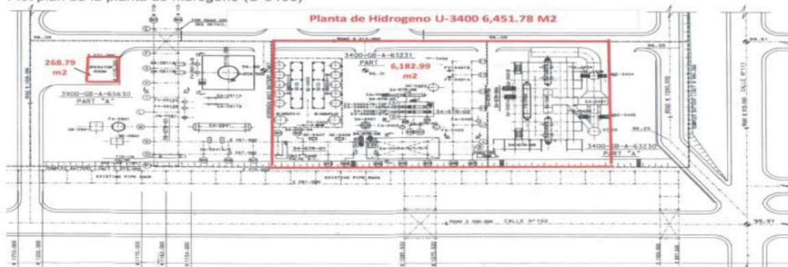
Plot plan de la planta de hidrógeno (U-3400)
