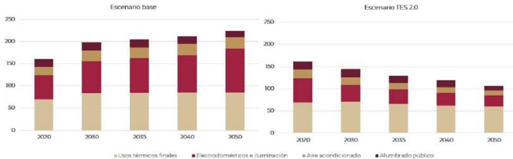
FIGURA 61 CONSUMO FINAL DE ENERGÍA DEL SECTOR COMERCIAL Y SERVICIOS 2020-2050, AMBOS ESCENARIOS (Petajoules)
