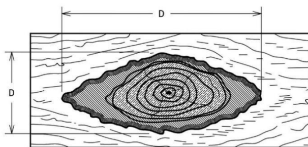
Figura 4 Nudo muerto
