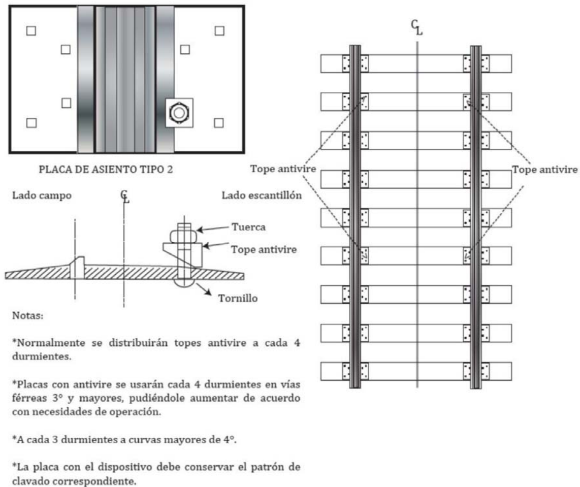
Figura 4 Dispositivos antivire.
