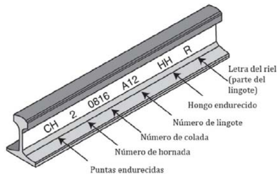
Figura 2 Marcado recomendable del lado interior del riel.
