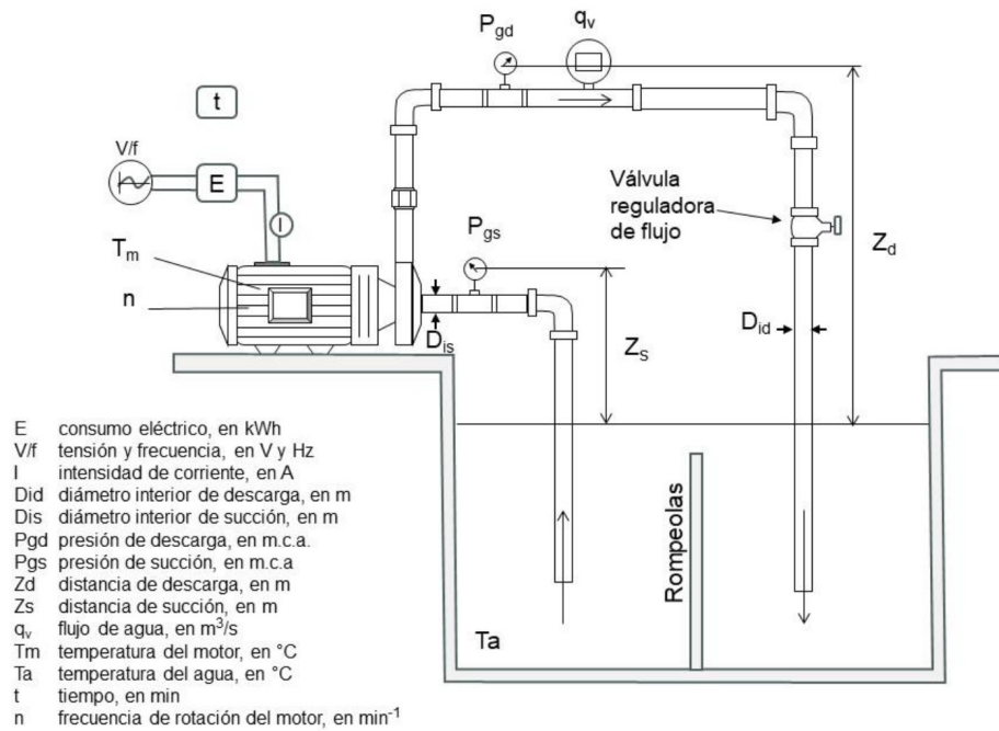
Figura A.2a - Arreglo sugerido para pruebas de estabilización y de comportamiento
